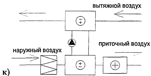
Рисунок Е.1 – Схемные решения утилизации теплоты удаляемого вентиляционного воздуха с УТ разных типов: а - рекуперативные ТО; б, в – калориферы; г – вращающиеся регенераторы; д – стационарные переключающиеся регенераторы; е – ТО с тепловыми трубками; ж – ТО с промежуточным теплоносителем; и, к – тепловые насосы
