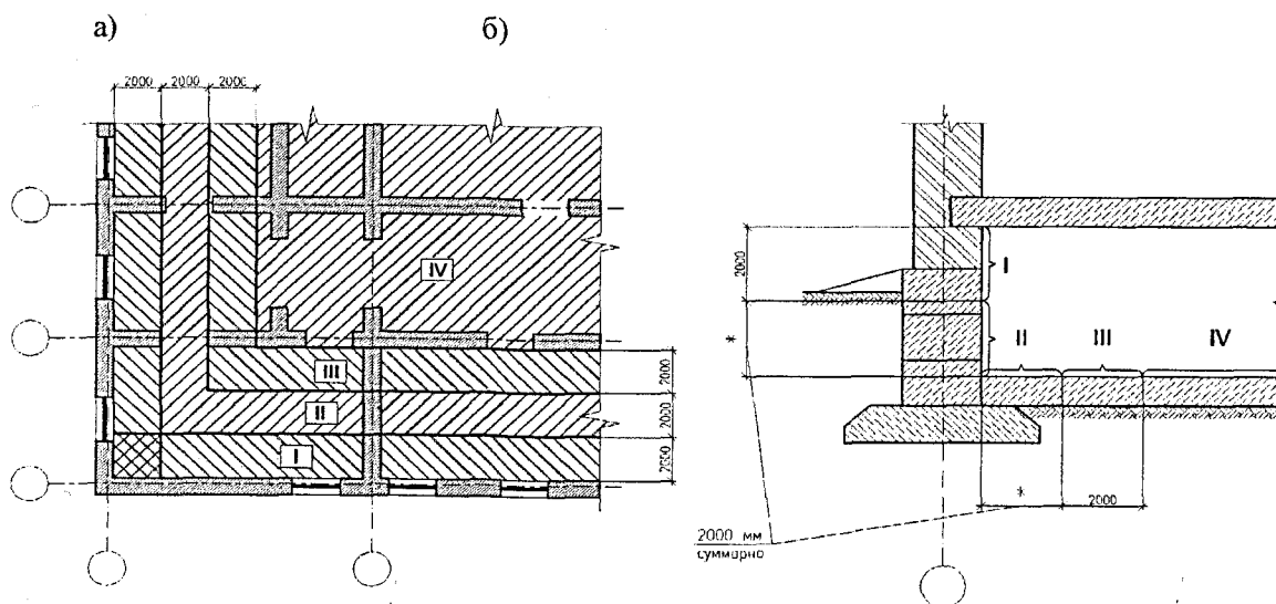
Рисунок Р.1 – Распределение поверхности пола (а) и заглубленных частей наружных стен (б), контактирующих с грунтом, по расчетным зонам I–IV
