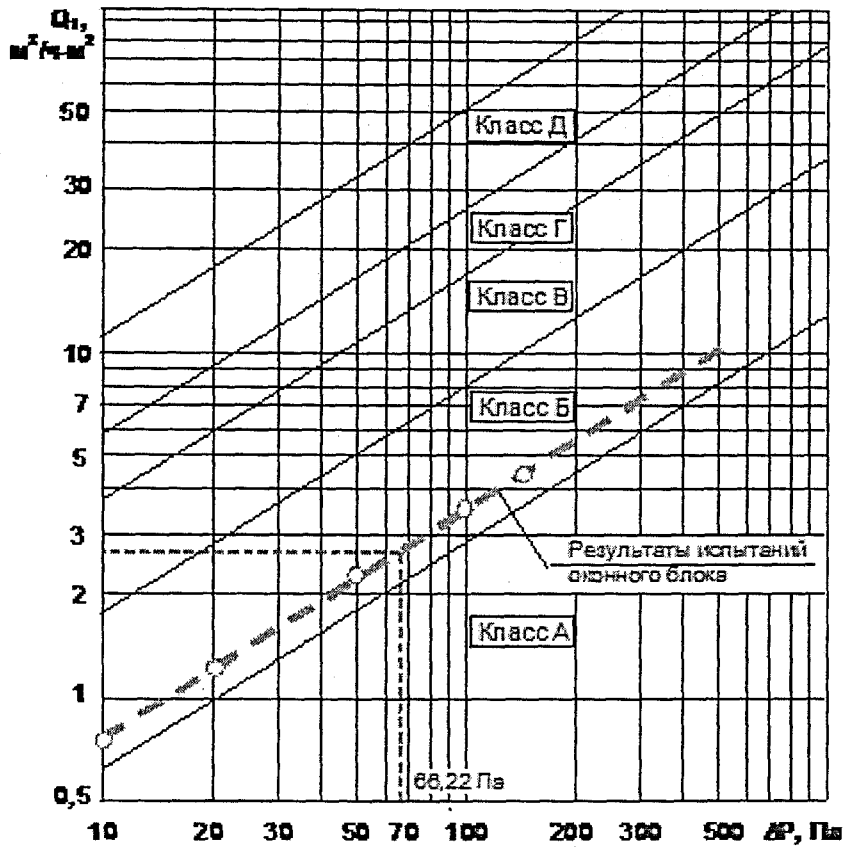
Рисунок С.2 –Зависимость объемной воздухопроницаемости оконного блока № 2 от перепада давления по результатам испытаний согласно ГОСТ 26602.2
