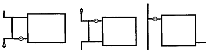
Рисунок Д.17 – Схемы установки термостатических головок на приборах СО
