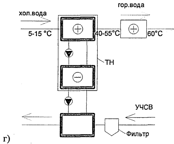
Подогрев воды для ГВС
