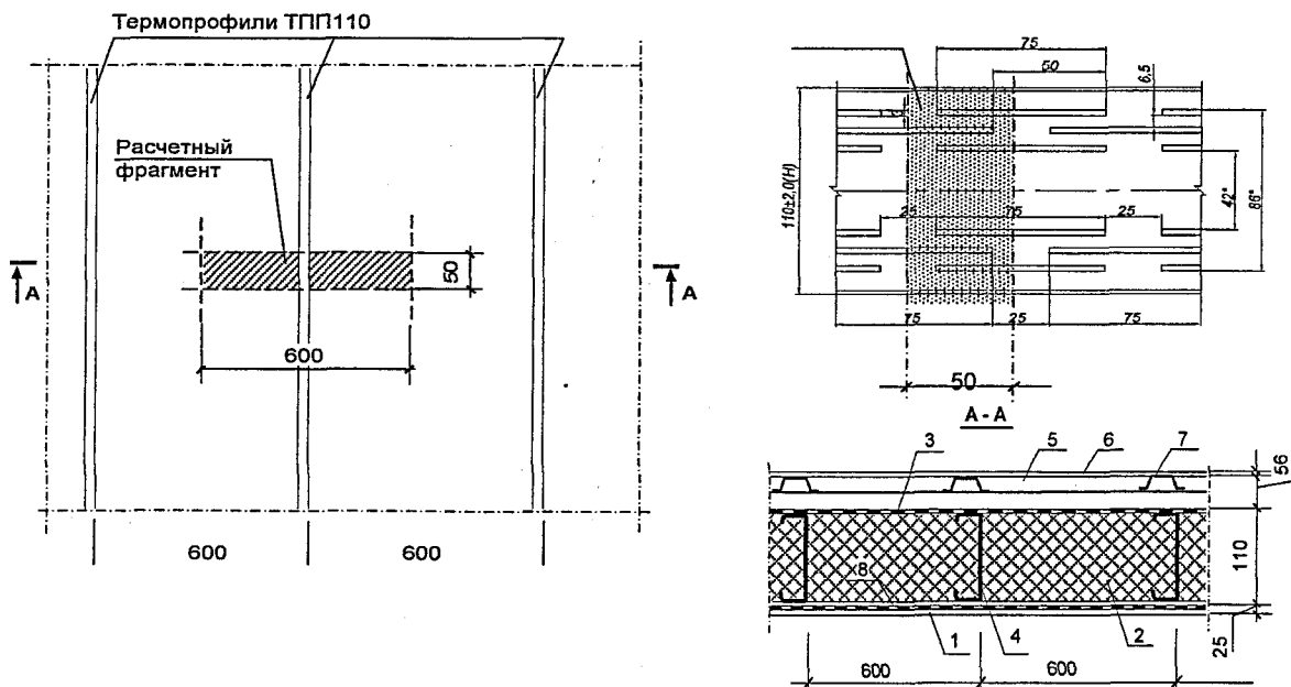
Рисунок Н.5 – Схема наружной стены с применением термопрофилей ТПП 110 к примеру Н.1 : 1 – внутренняя обшивка; 2 – утеплитель; 3 – гидро-ветрозащита; 4 – термопрофиль ТПП 110; 5 – вентилируемая воздушная прослойка; 6 – наружная облицовка; 7 – шляпный профиль; 8 – пароизоляция
