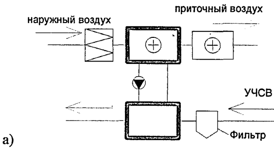
Подогрев холодной воды в холодный период года
