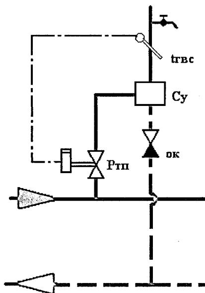
Рисунок Д.11 – Схема автоматизации подготовки горячей воды для открытой системы ГВС
