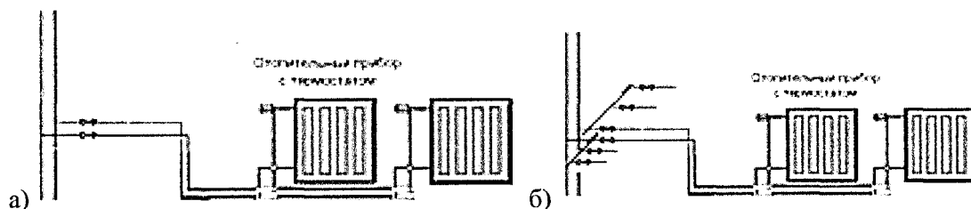
Рисунок Д.5 – Подключение внутриквартирных систем к стоякам:
