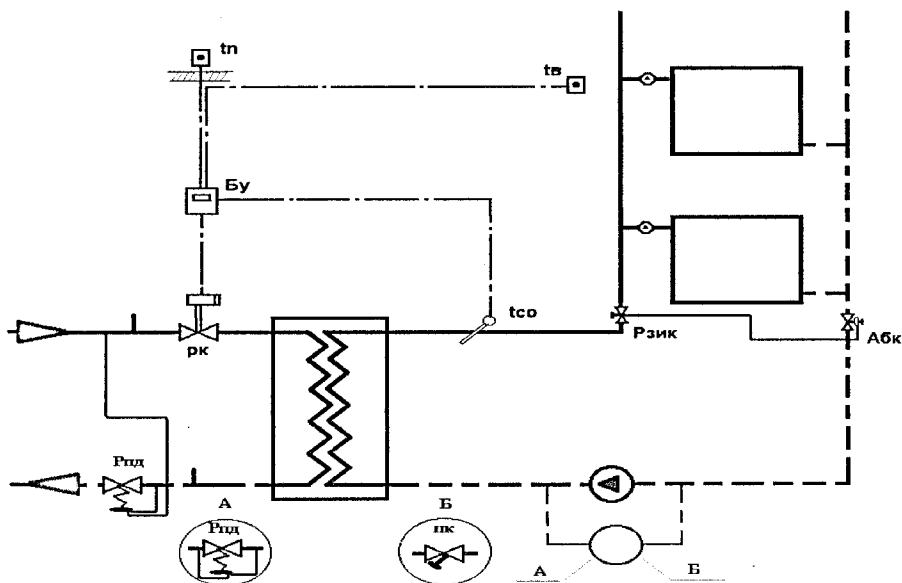
Рисунок Д.10 – Схема автоматизация теплового пункта с независимым присоединением СО
