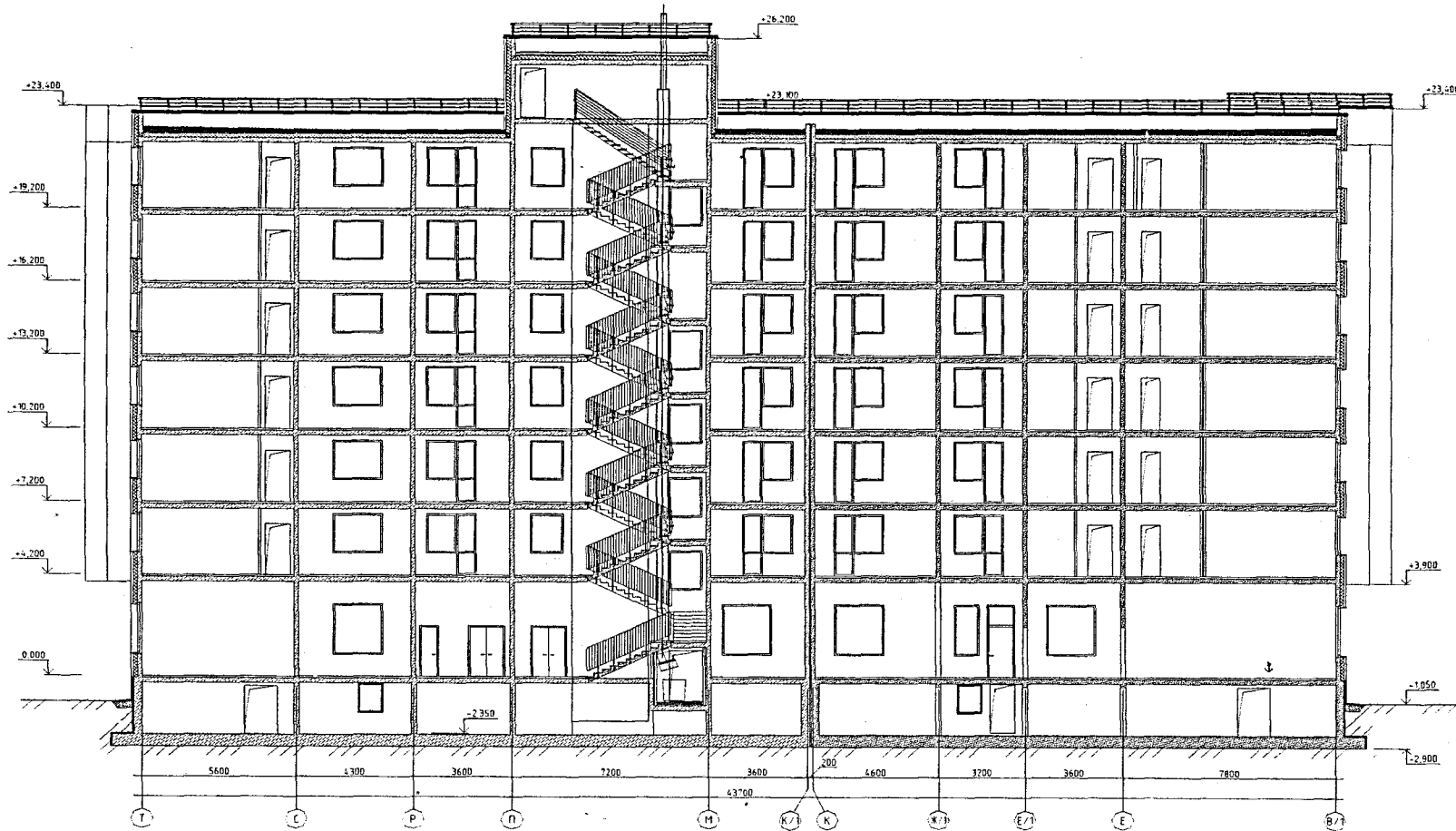
Рисунок Т.4 – Разрез здания в осях Т-В/1
