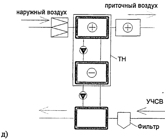
Нагрев приточного воздуха
