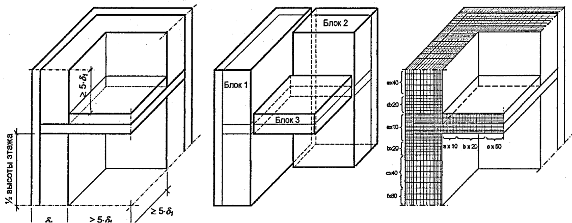
Рисунок Н.3 – Примеры разбиения расчетной области на конечные элементы: а – для расчета двухмерного температурного поля; б – для расчета трехмерного температурного поля
