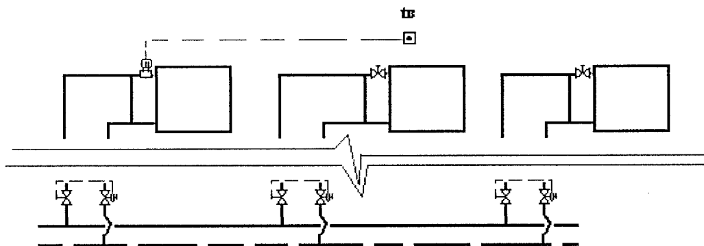
Рисунок Д.2–Схема установка термостатов в двухтрубных системах отопления
