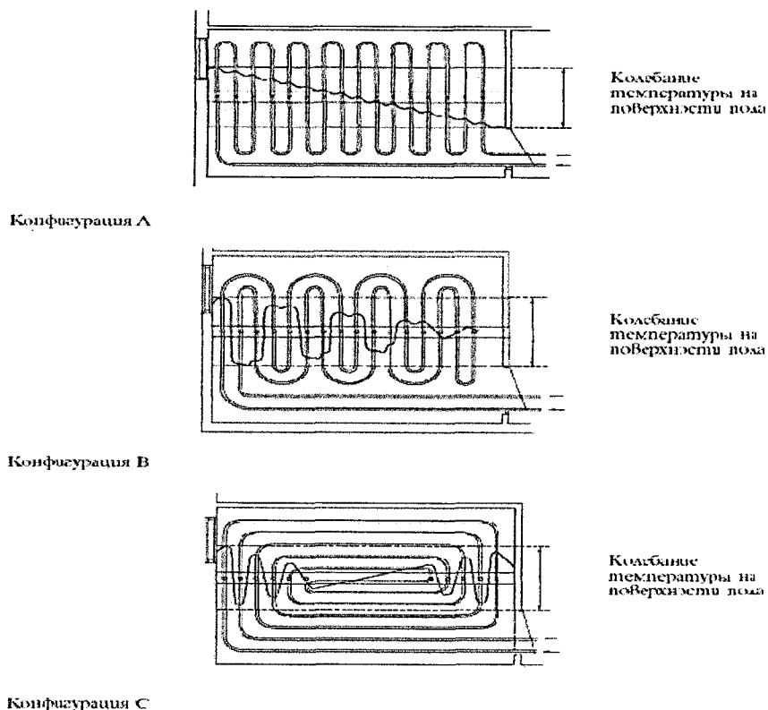
Рисунок Д.6–Раскладка греющих контуров системы напольного отопления
