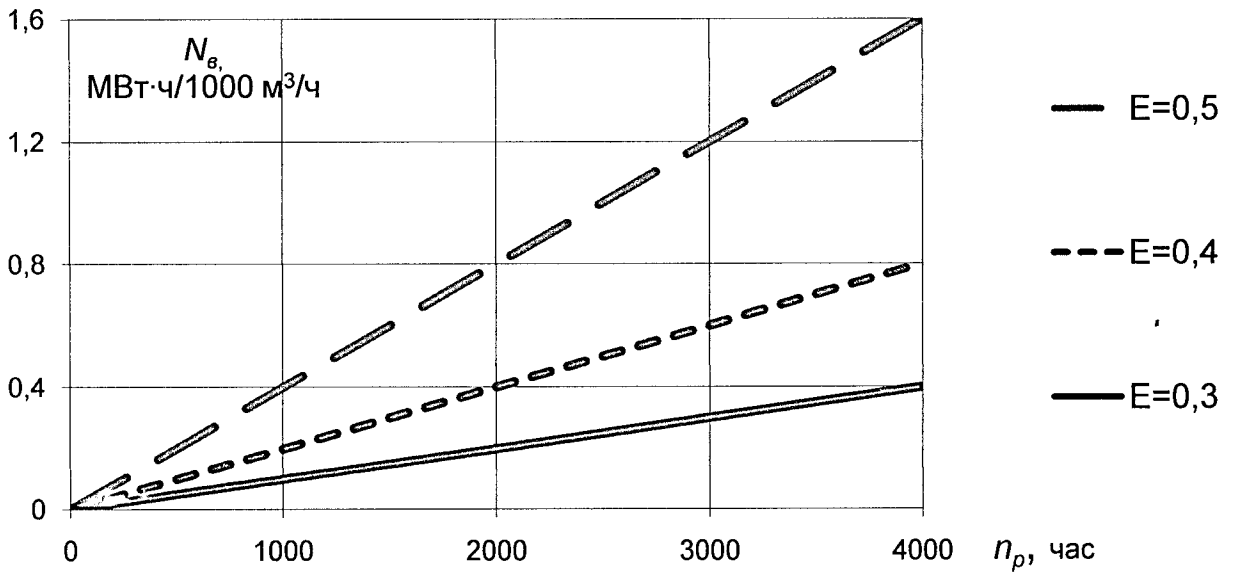
Рисунок Е.5 – Зависимость дополнительного годового расхода электроэнергии от числа часов и степени утилизации теплоты
