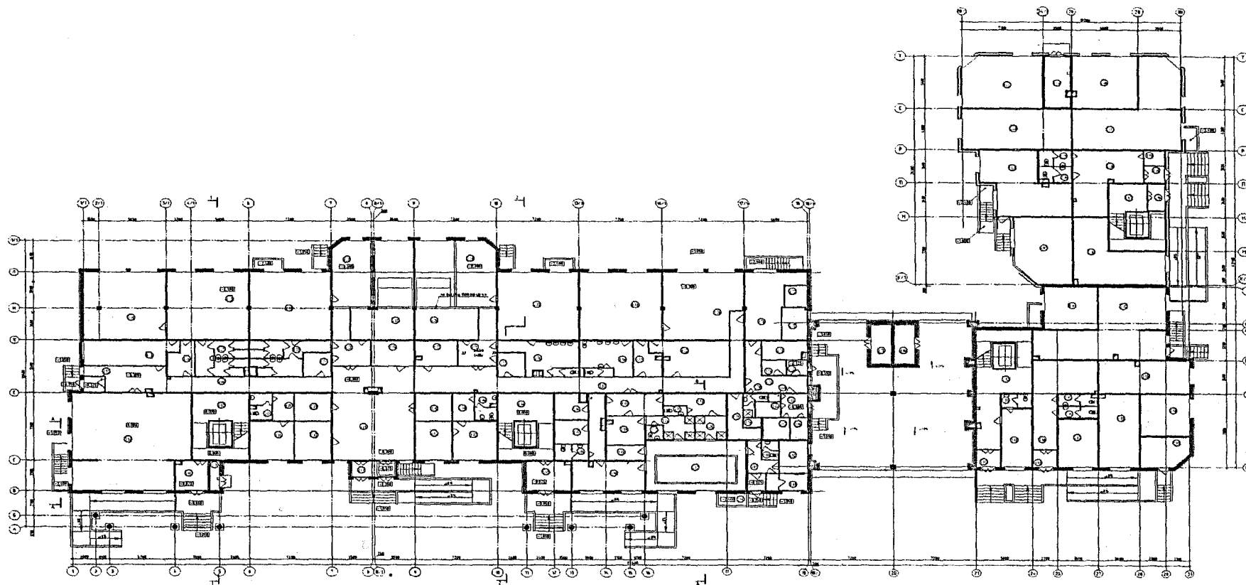
Рисунок Т.2 – План первого этажа здания
