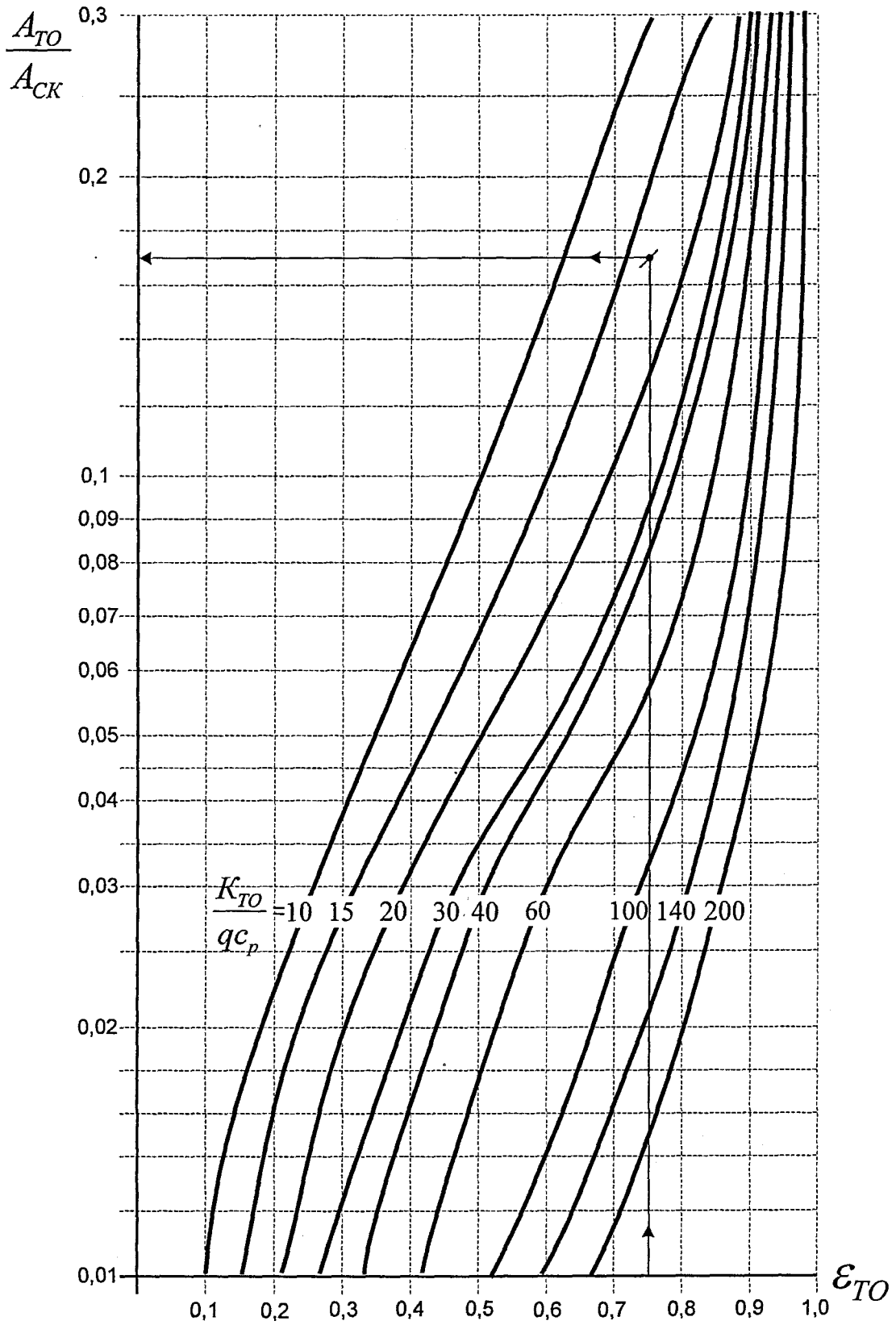
Рисунок Е.15 – График определения относительной площади теплообменника
