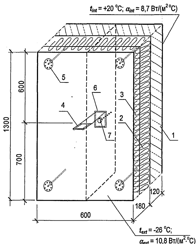
Рисунок Н.8 – Расчетная схема (а) и результаты расчета распределения температур (б) по сечению стены в зоне расположения кронштейна:
