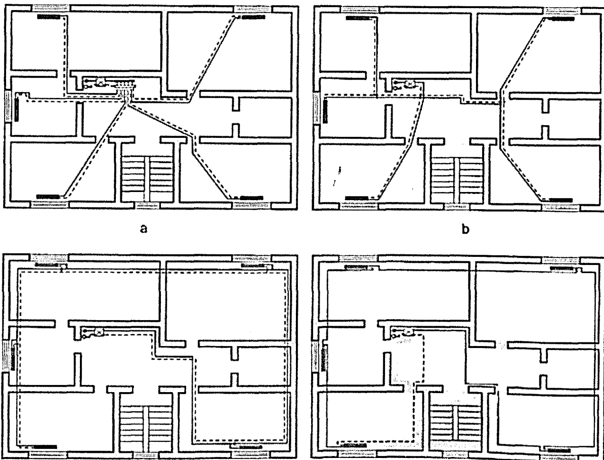
Рисунок Д.4 – Варианты схемных решений поквартирной разводки: а) лучевая с распределительным коллектором; б) лучевая бесколлекторная; в) кольцевая двухтрубная; г) кольцевая однострунная
