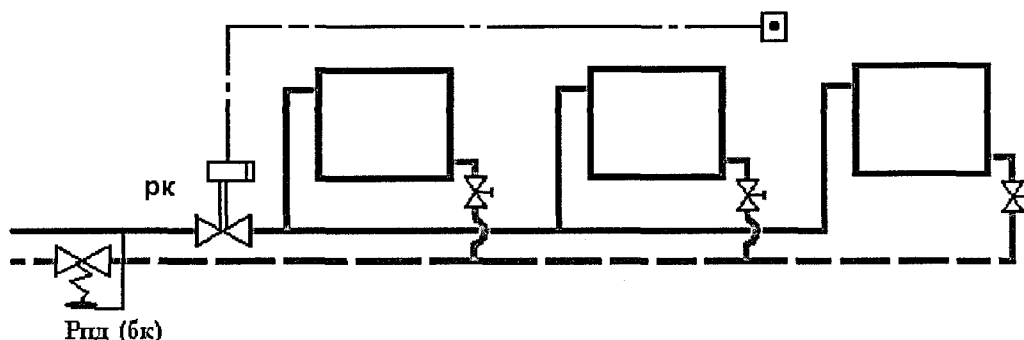
Рисунок Д.16 – Схема автоматизации горизонтальных СО
