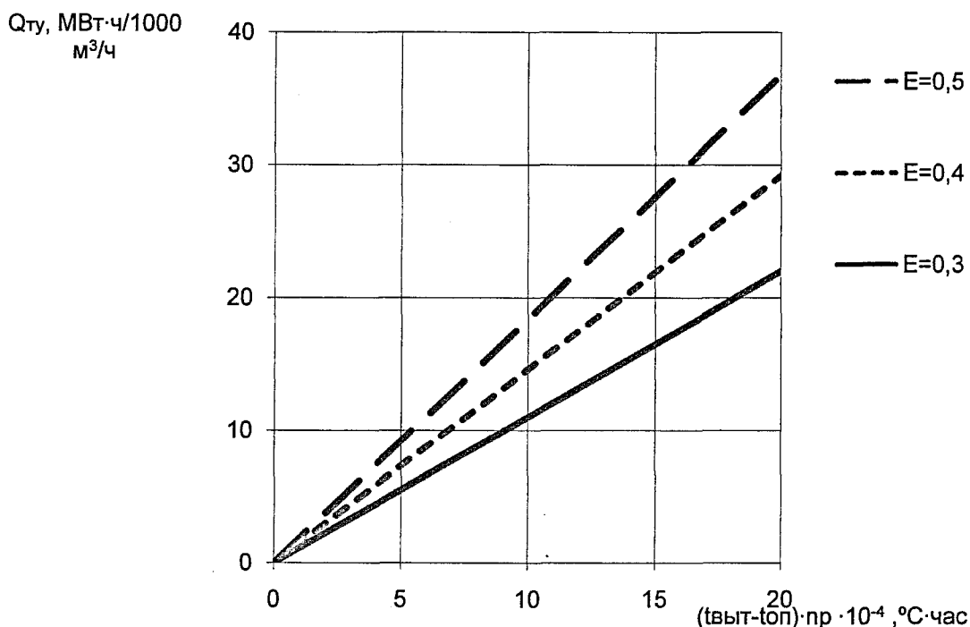
Рисунок Е.3 – Зависимость годовой экономии теплоты от градусо-часов работы и степени утилизации теплоты
