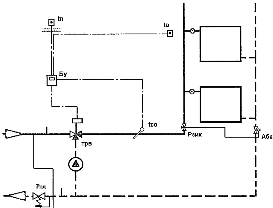
Рисунок Д.9 – Схема автоматизация теплового пункта с зависимым присоединением СО
