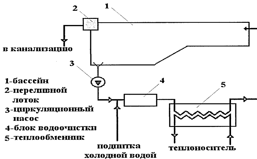
Рисунок Е.6 –Принципиальная схема оборотного водоснабжения бассейна
