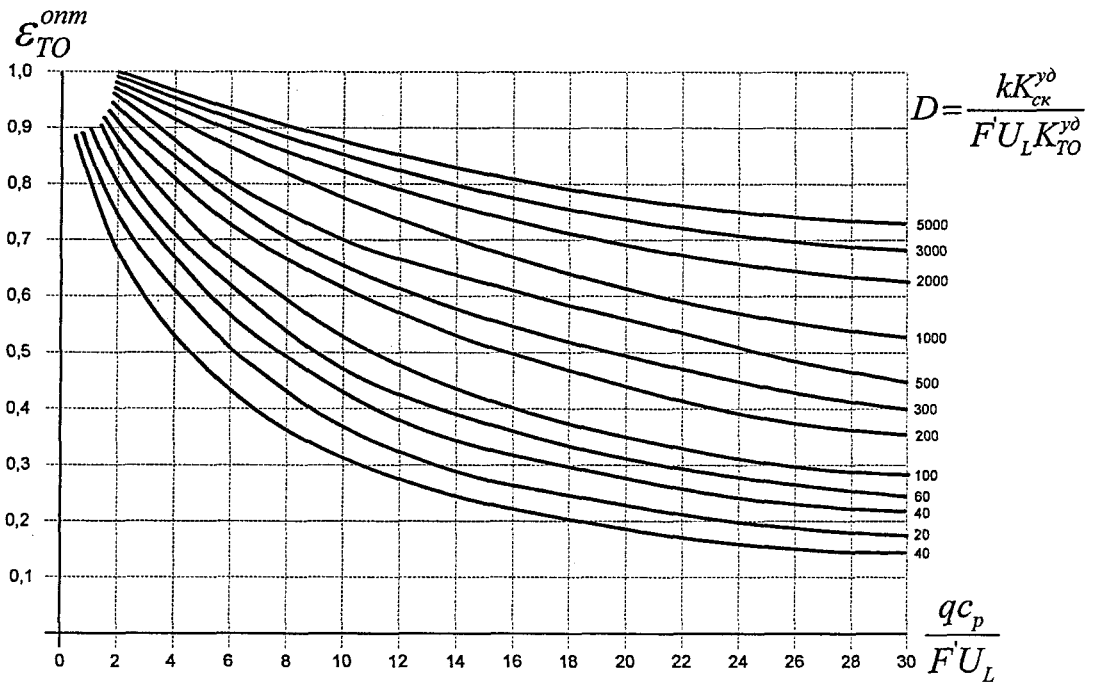
Рисунок Е.14 – График определения значения эффективности теплообменника
