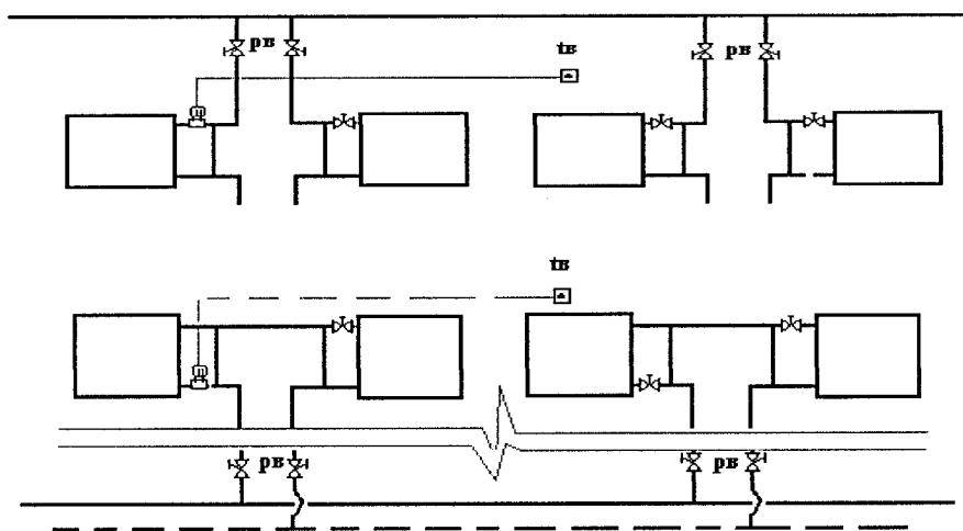
Рисунок Д.1 – Схема установка термостатов в однотрубных системах отопления
