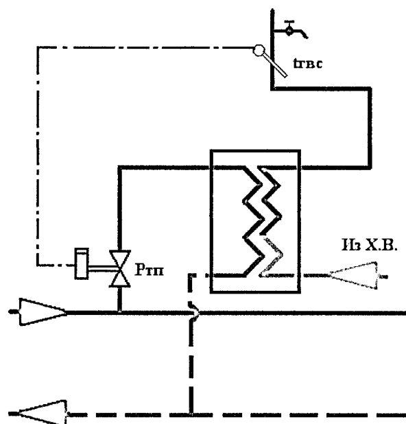
Рисунок Д.12 – Схема автоматизации подготовки горячей воды для закрытой системы ГВС
