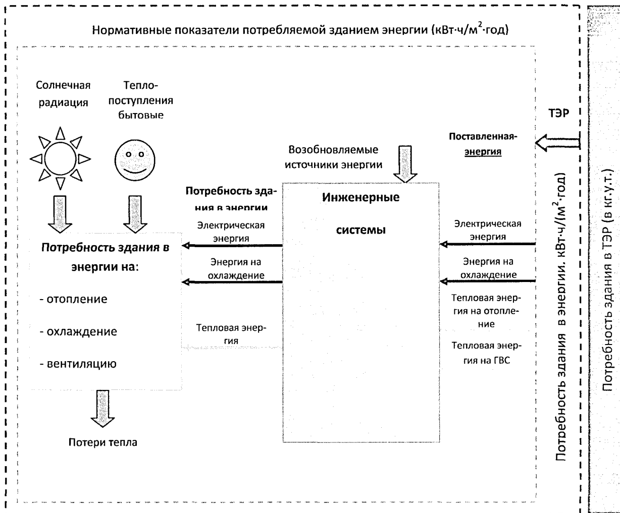
Рисунок 1 – Схема годового баланса потребления зданиями ТЭР
