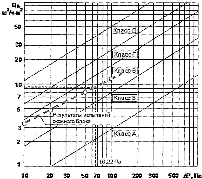
Рисунок С.1 – Зависимость объемной воздухопроницаемости оконного блока № 1 от перепада давления по результатам испытаний согласно ГОСТ 26602.2
