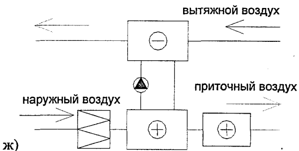
Нагрев (и охлаждение при реверсивном ТН) приточного воздуха
