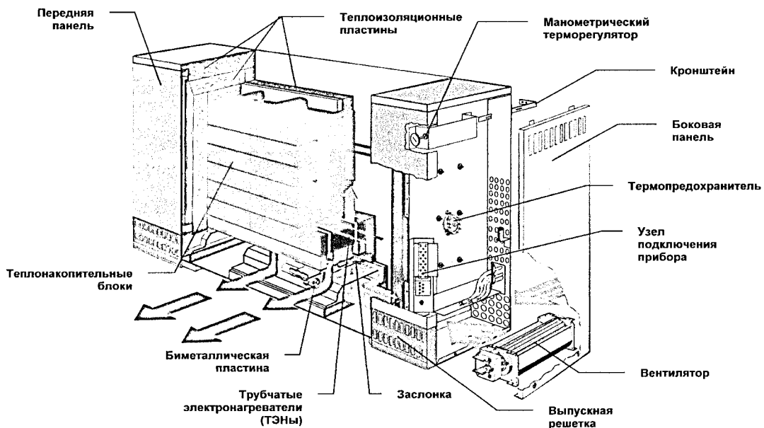
Рисунок Д.8–Принципиальная схема теплоинерционного отопительного прибора
