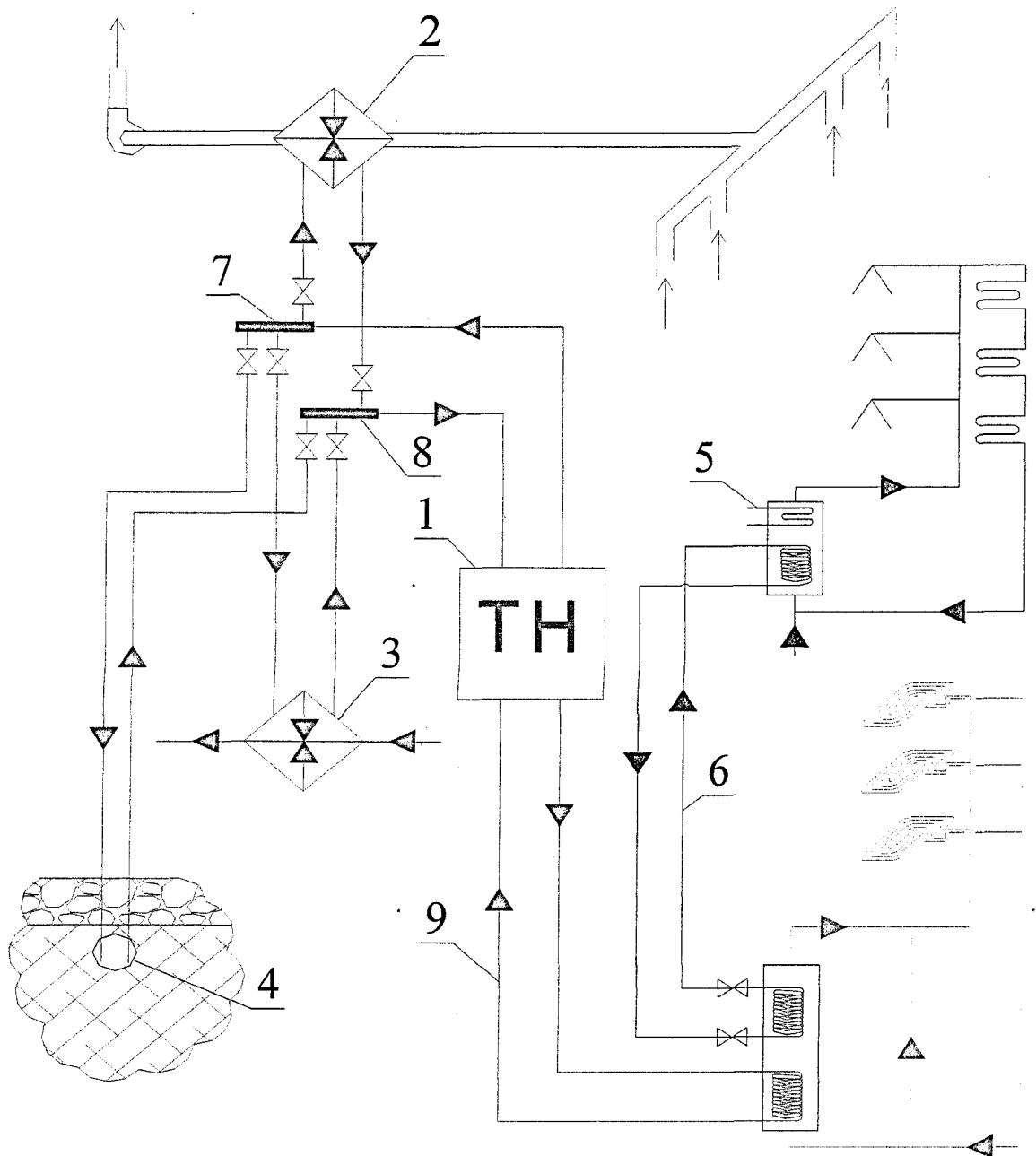
Рисунок Е.9 – Принципиальная схема (избыточная) теплонасосной системы теплоснабжения здания с использованием собственных ИНТ: 1 – тепловой насос; 2, 3, 4 – теплообменники системы теплосбора (соответственно, удаляемого вентиляционного воздуха, условно чистых сточных вод, грунта); 5 – дублирующий источник теплоты (догреватель) ГВС; 6 – промежуточный контур ГВС; 7, 8 – коллекторы (гребенки) первого контура ТНУ; 9 – второй контур ТНУ.
