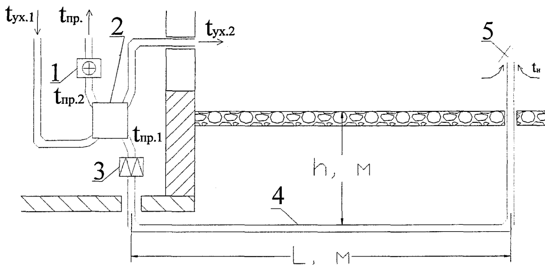
Рисунок Е.17 – Принципиальная схема вентиляции здания с утилизацией теплоты грунта и вытяжного воздуха: 1 – пиковый догреватель; 2 – утилизатор теплоты; 3 – фильтр; 4 – грунтовый теплообменник; 5 – воздухозаборный оголовок
