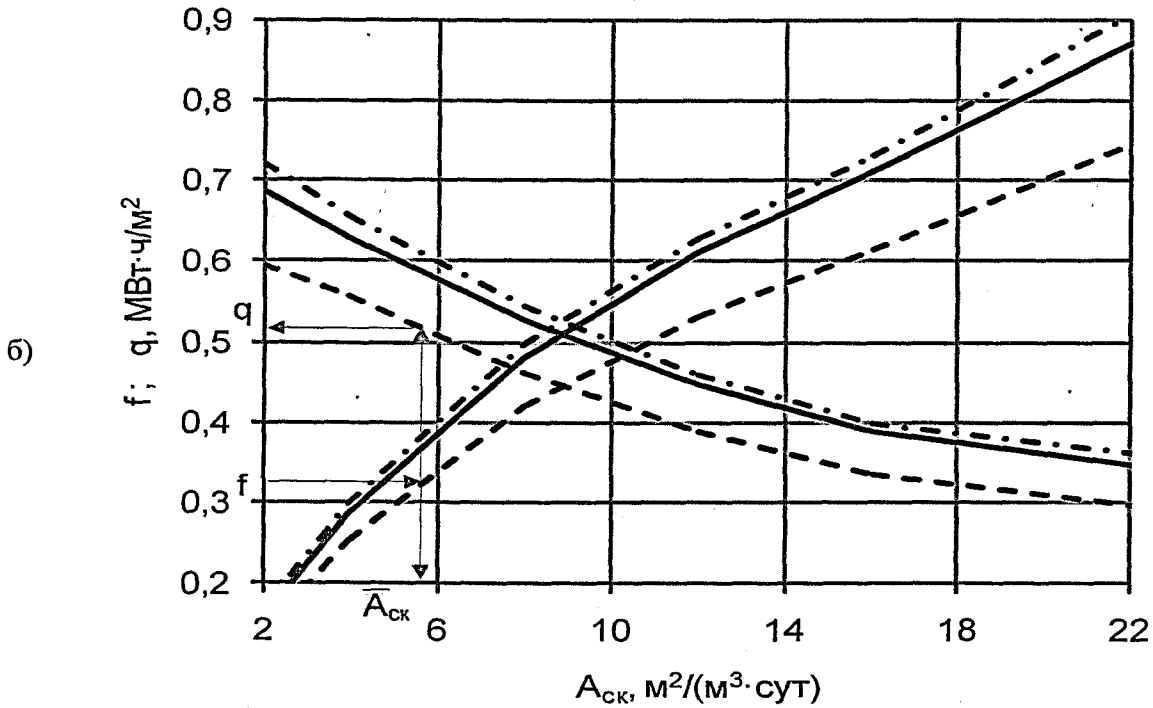
Рисунок Е.13 – Графики для определения удельной площади и годовой выработки теплоты: а) при температуре горячей воды 55°С; б) при температуре горячей воды 30°С
