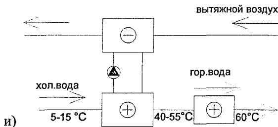
Подогрев воды для ГВС
