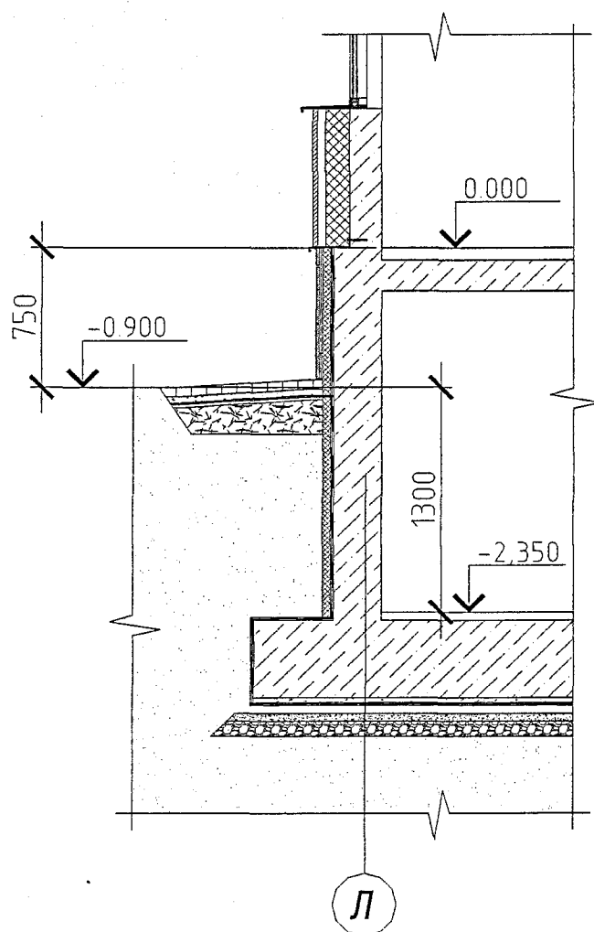
Рисунок Л.1 – Разрез ограждающих конструкций техподполья ниже уровня пола здания
