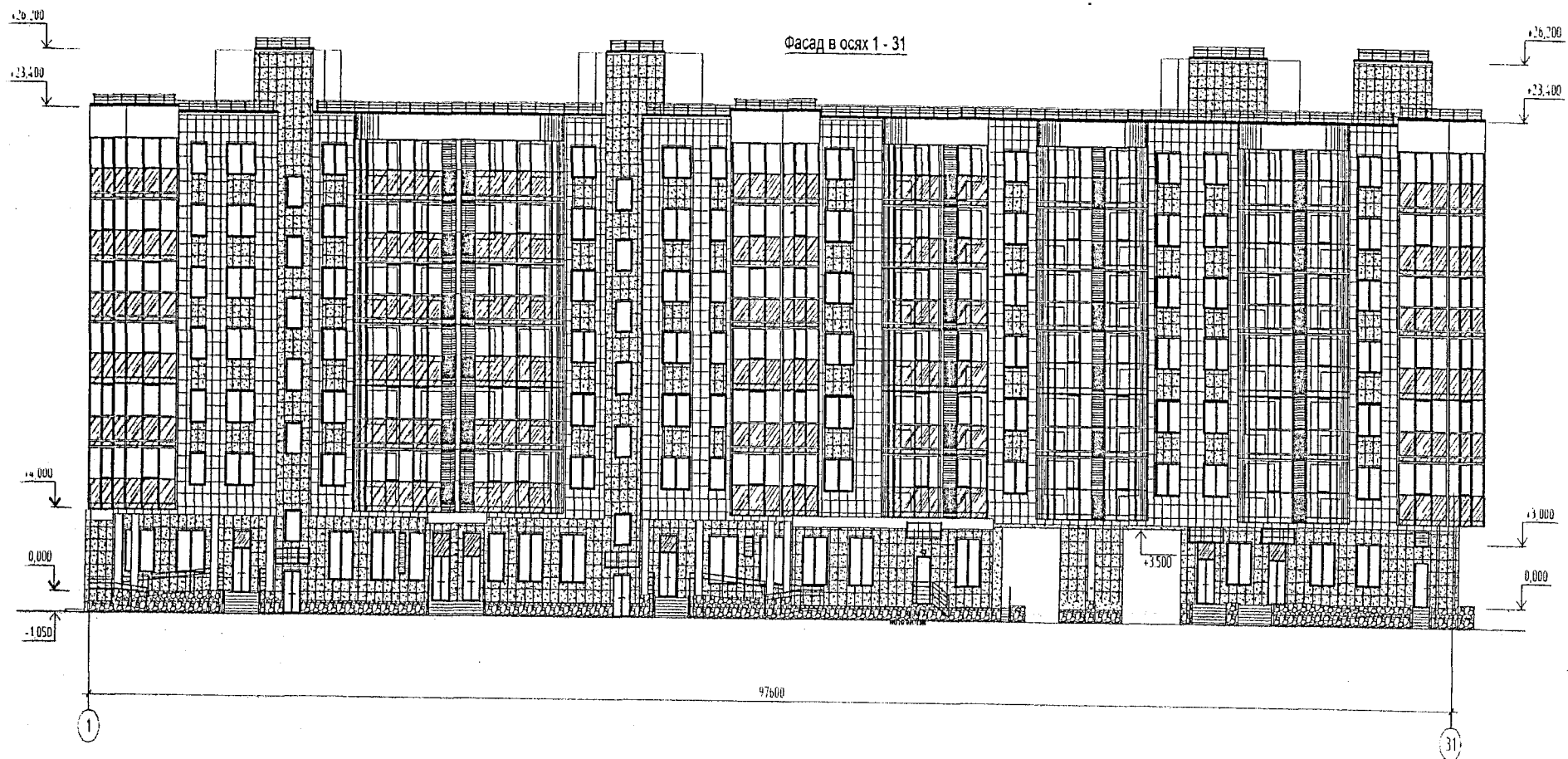
Рисунок Т.1 – Фасад в осях 1–31
