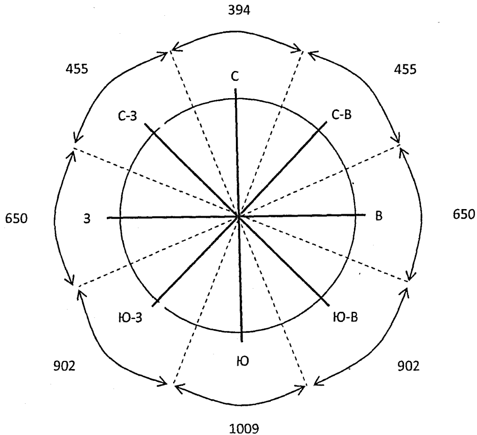
Рисунок Ц.1 – Распределение средней величины солнечной суммарной радиации на вертикальные поверхности при действительных условиях облачности I_{в,i} , MДж/m^2 , за отопительный период для климатических условий Санкт-Петербурга
