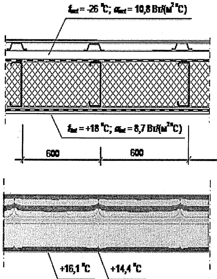
Рисунок Н.6 – Расчетная схема (а) и результаты расчета распределения температур (б) по сечению стены
