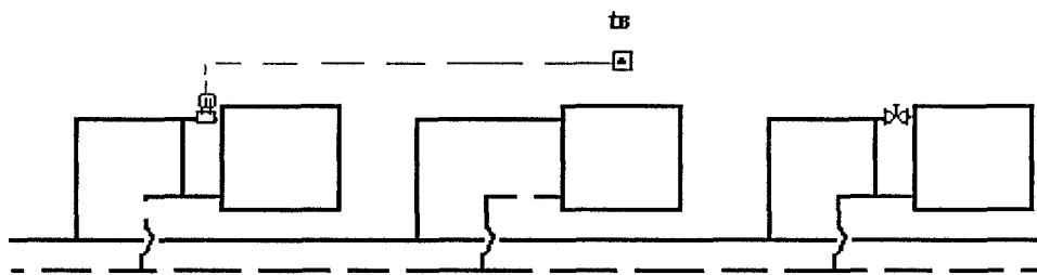
Рисунок Д.3 – Схема установка термостатов в горизонтальных системах отопления
