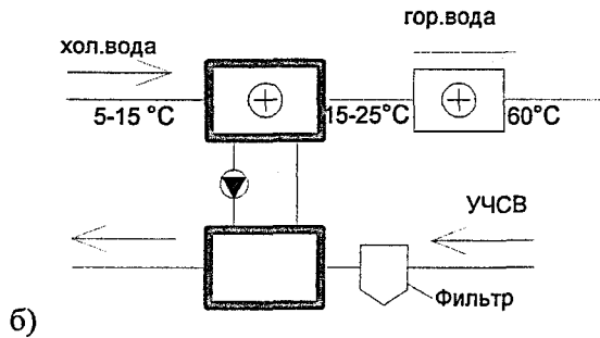
Подогрев воды для ГВС
