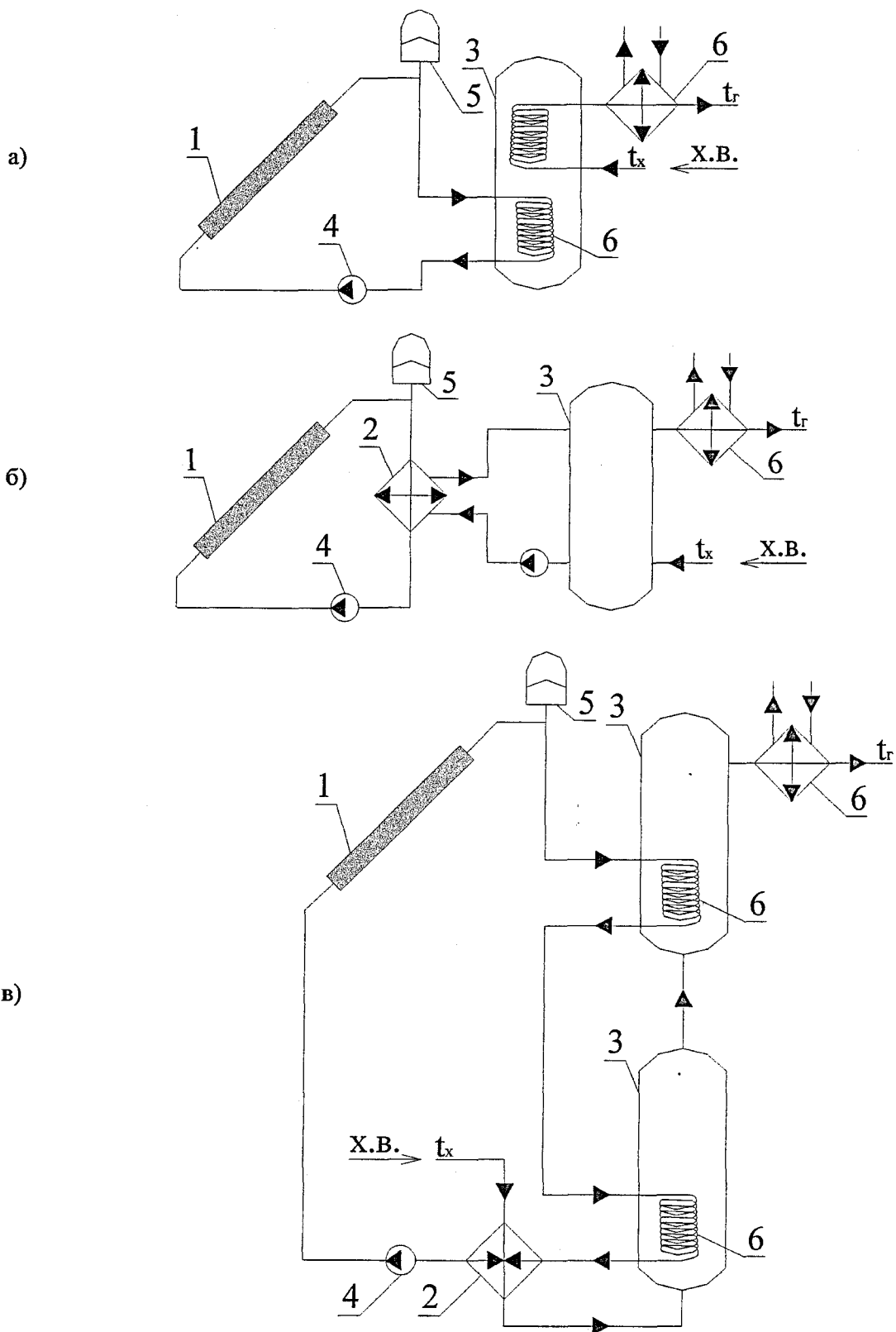
Рисунок Е.12 – Принципиальная схема двухконтурной гелиосистемы: 1 – солнечный коллектор; 2 – промежуточный теплообменник; 3 – бак-аккумулятор; 4, 7 – циркуляционные насосы; 5 – расширительный бак; 6 – дублирующий источник теплоты (догреватель)
