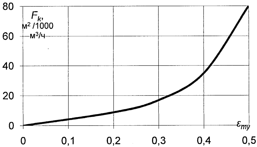
Рисунок Е.4 – Зависимость площади теплопередачи caloriferов–теплоутилизаторов от степени утилизации \epsilon_{\mu}
