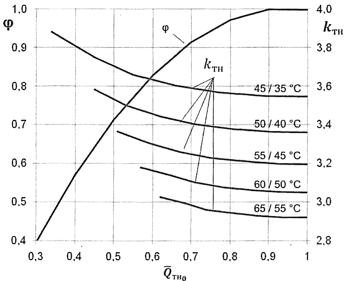
Рисунок Е.11 – Графики зависимости годового коэффициента замещения отопительной нагрузки и среднего коэффициента преобразования от относительной теплопроизводительности ТНУ и расчетных температур теплоносителя в системе отопления для грунтовой системы теплосбора
