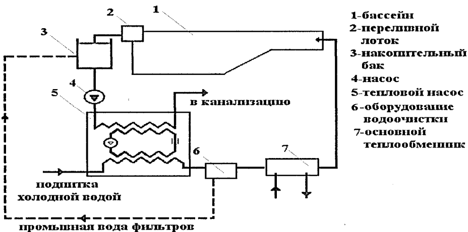
Рисунок Е.8 – Утилизация теплоты сбрасываемых вод с помощью теплового насоса
