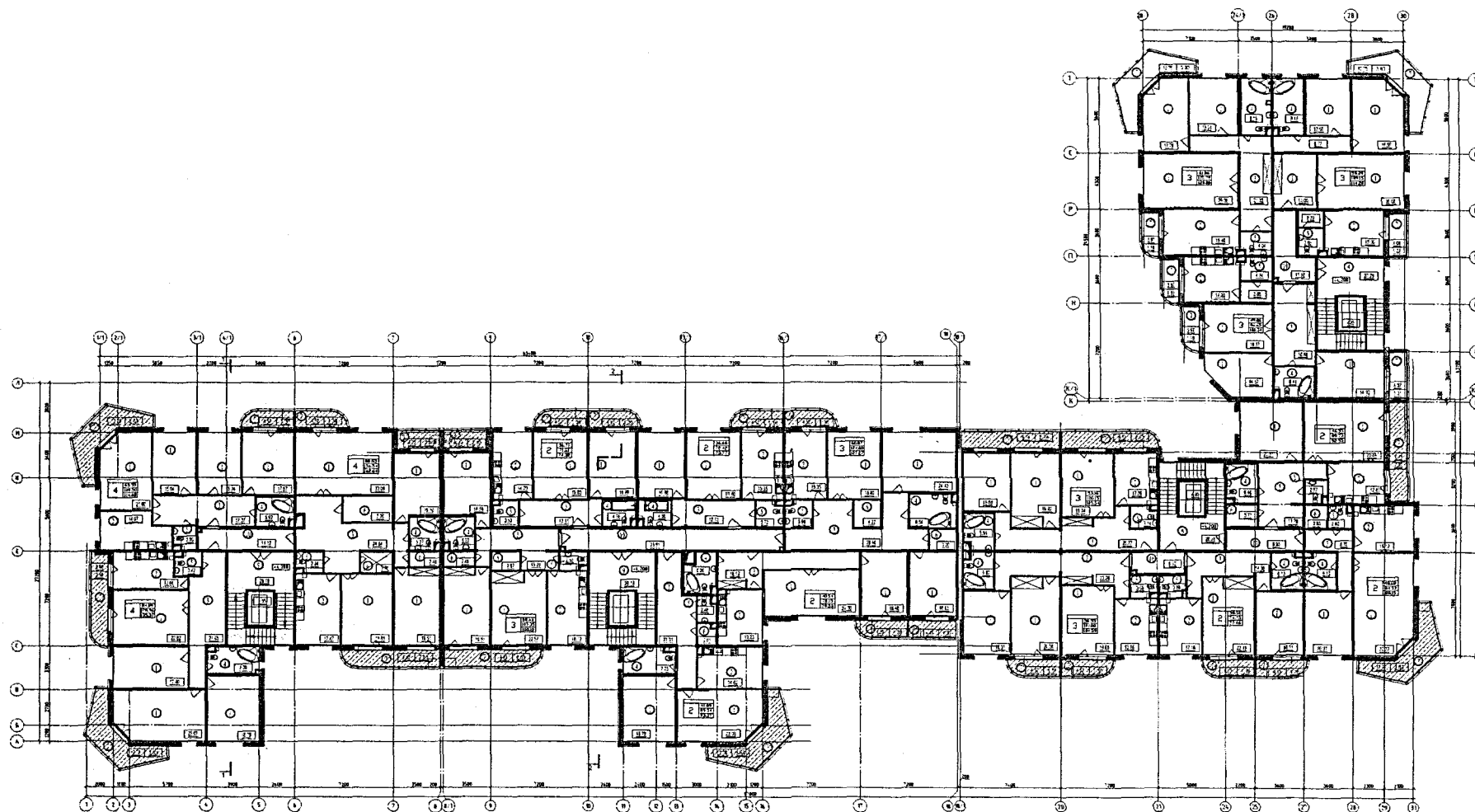
Рисунок Т.3 – План второго (типového) этажа здания
