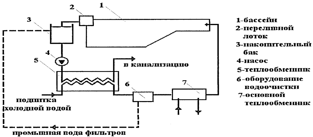
Рисунок Е.7 – Утилизация теплоты сбрасываемых вод с помощью теплообменника
