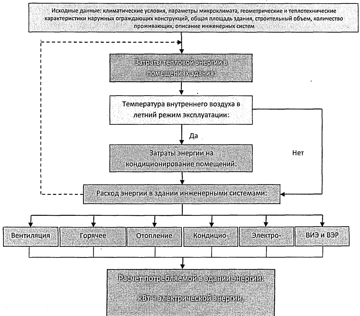
Рисунок Ю.1 – Блок-схема последовательности расчета расхода потребляемой энергии
