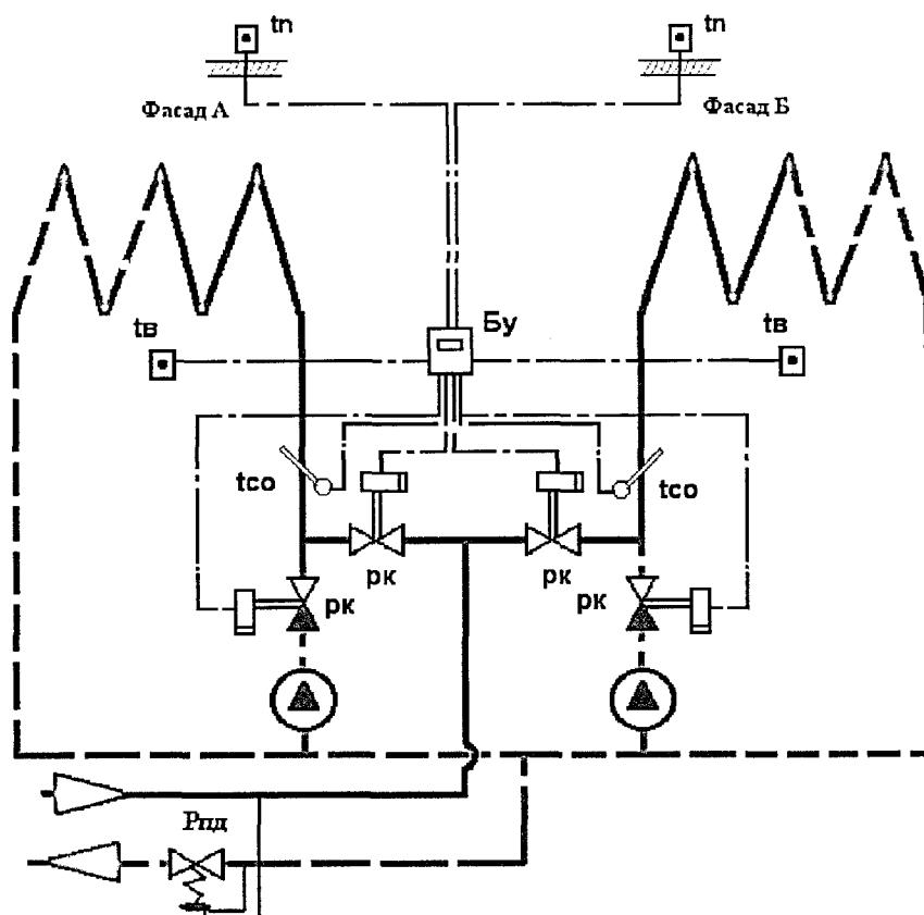
Рисунок Д.14 – Схема пофасадной автоматизации при зависимом подключении СО
