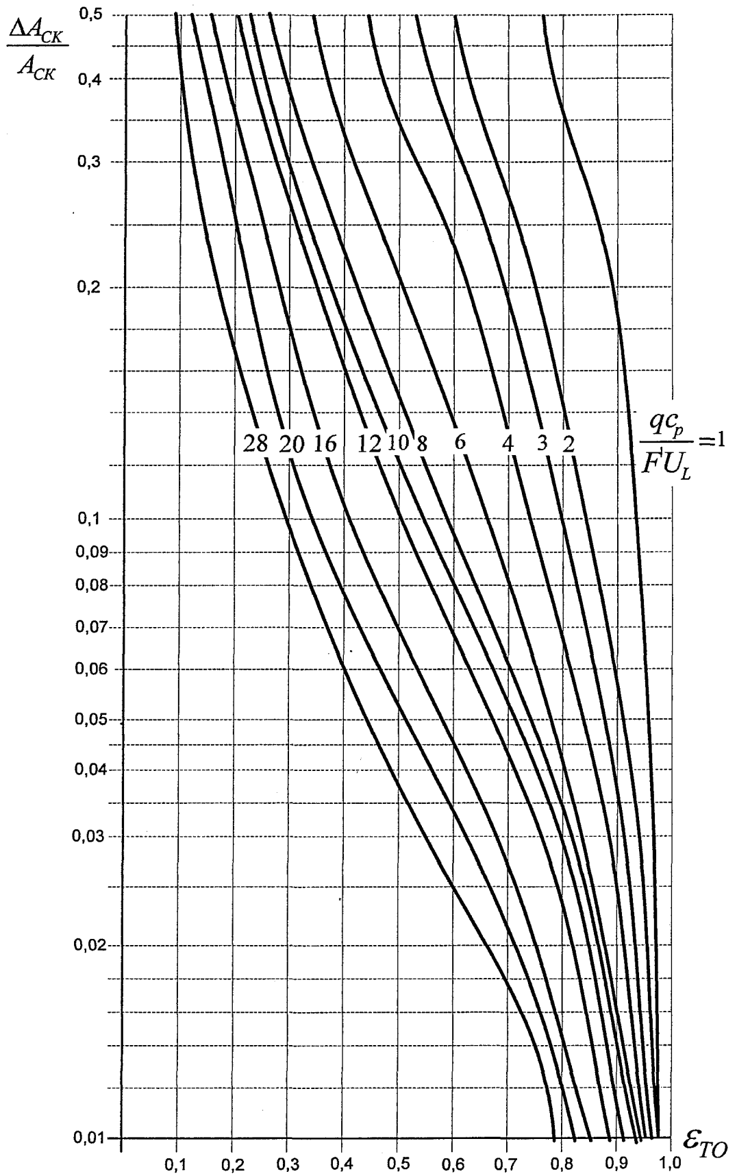
Рисунок Е.16 – Относительное увеличение площади солнечных коллекторов
