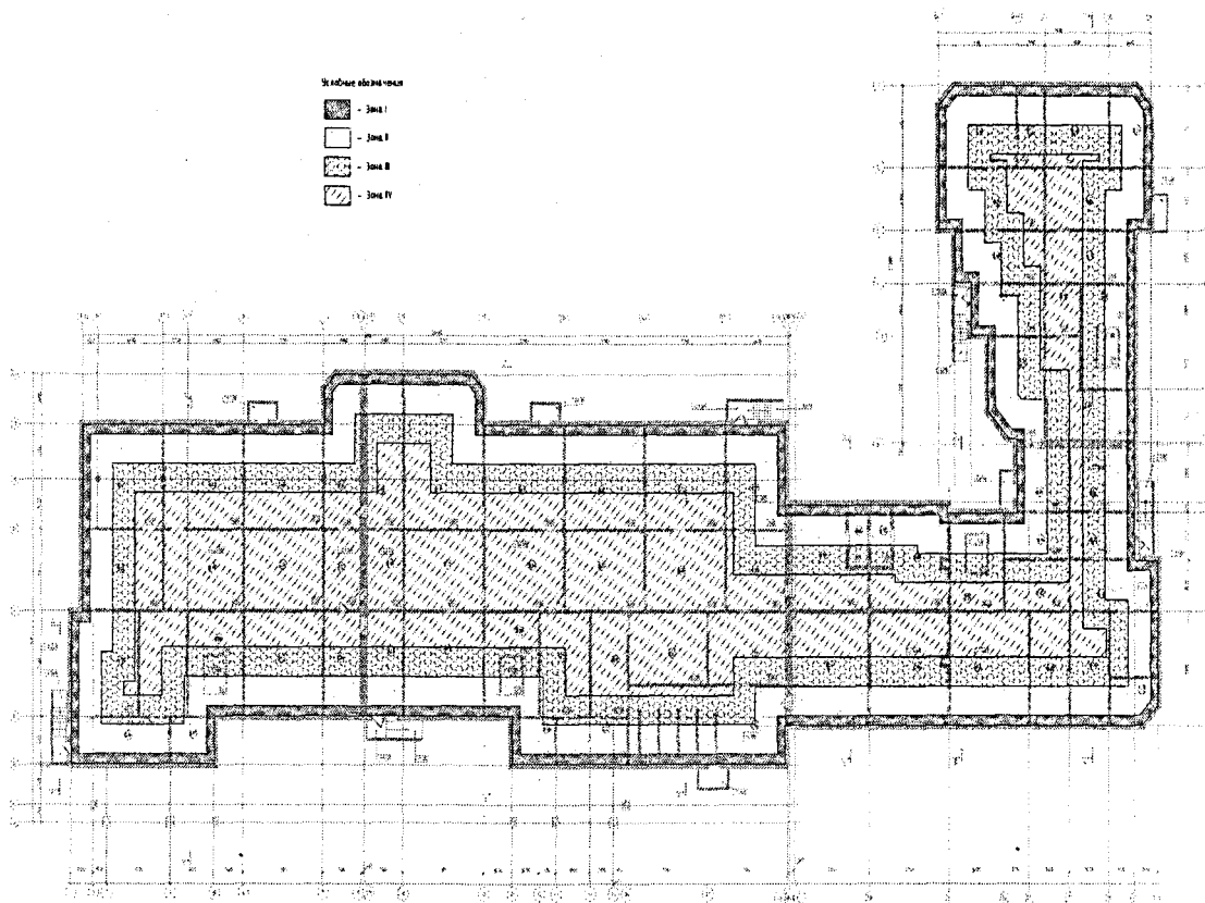
Рисунок Р.2 – План техподполья здания по зонам
