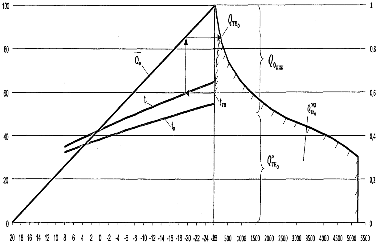
Рисунок Е.10 – К определению основных характеристик теплонасосного отопления
