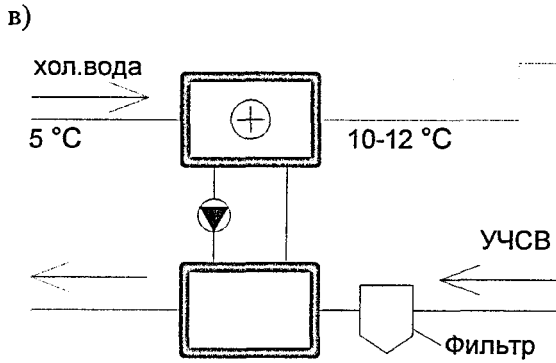
Подогрев холодной воды в холодный период года
