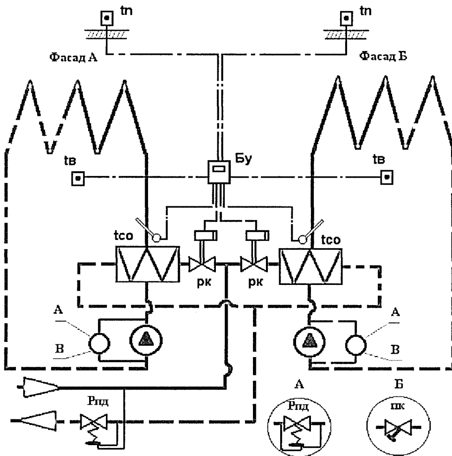
Рисунок Д.15 – Схема пофасадной автоматизации при независимом подключении СО
