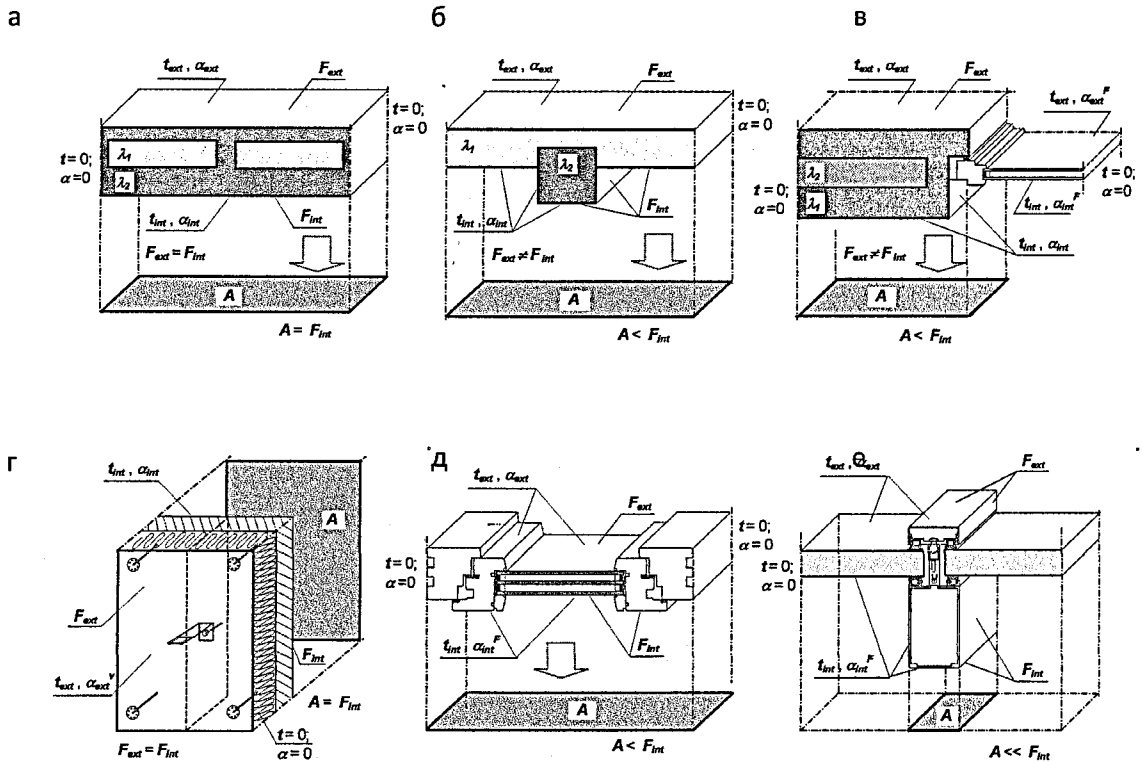
Рисунок Н.4 – Примеры задания граничных условий и определения площадей приведения A_i для расчета приведенного сопротивления теплопередаче некоторых конструкций: а, б – фрагмента наружной стены с теплопроводными включениями без проемов; в – фрагмента наружной стены с оконным блоком; г – фрагмента наружной стены с фасадной изоляцией; д – оконного блока; е – системы профилей
