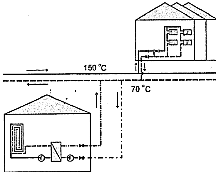
Рисунок Д.7 – Подключение здания к обратному трубопроводу тепловой сети
