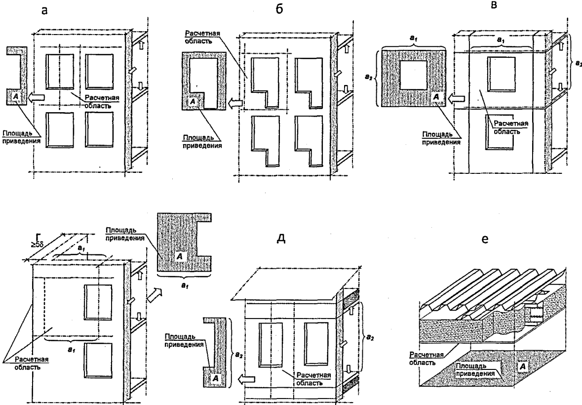
Рисунок Н.2 – Примеры выбора расчетной области для некоторых типов конструкций: а – стена с окнами; б – стена с балконными дверями; в – стеновая панель крупнопанельного здания; г – стена углового помещения; д – стена одноэтажного здания; е – совмещенное покрытие
