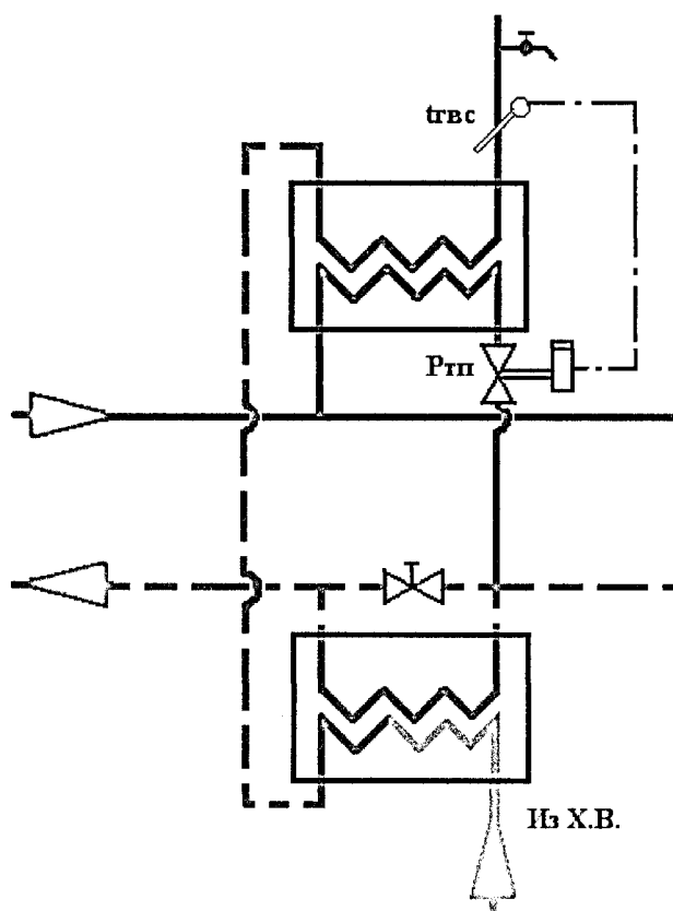
Рисунок Д.13–Схема автоматизации подготовки горячей воды для закрытой системы ГВС
