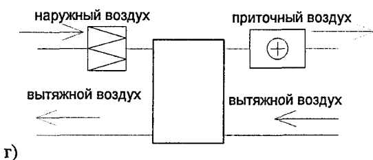
Нагрев (охлаждение) приточного воздуха
