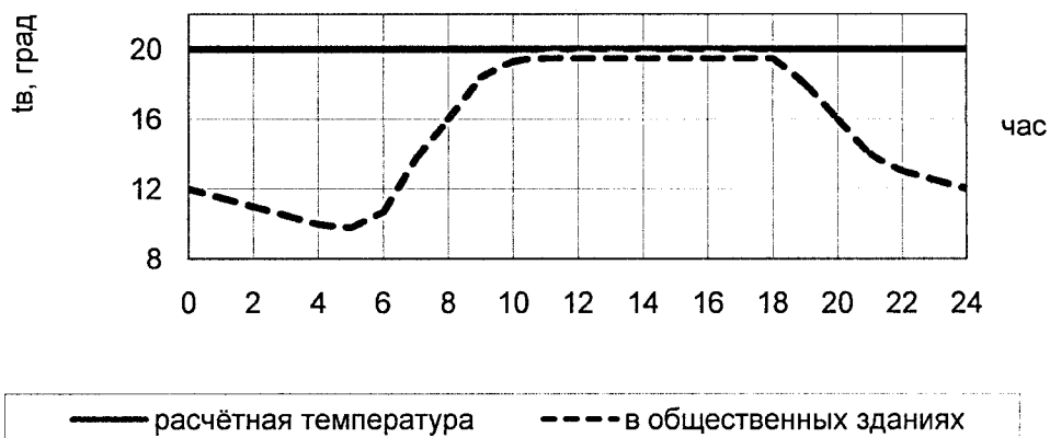
Рисунок Д.21 – Суточные режимы подачи тепла и соответствующие температурные режимы в жилых и общественных зданиях
