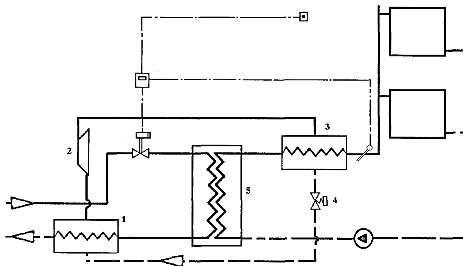
1 - испаритель; 2 - компрессор; 3 - конденсатор т.н.; 4 - редуктор; 5 - теплообменник системы отопления
