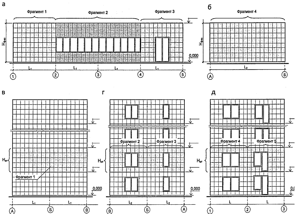
Рисунок Н.1 – Примеры разбиения фасада здания (а, б) или промежуточного этажа (в, г, д) на отдельные фрагменты для расчета приведенного сопротивления теплопередаче
