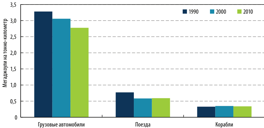
Рисунок 6.16 • Пример показателя уровня 2: энергопотребление на тонно-километр по видам транспорта
