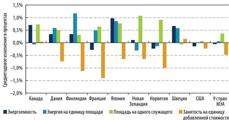
Рисунок 4.9 • Декомпозиция изменений в энергоемкости сектора услуг, 1990–2010 годы
