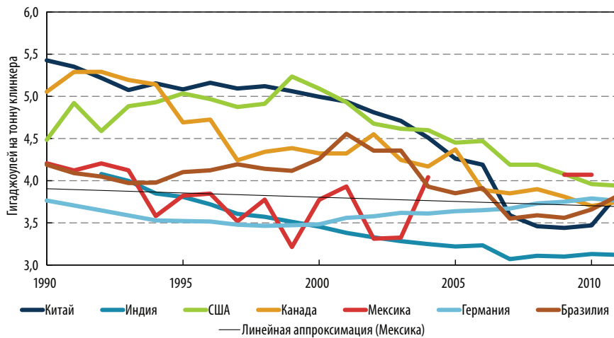
Рисунок 5.9 • Энергопотребление на тонну клинкера по странам
