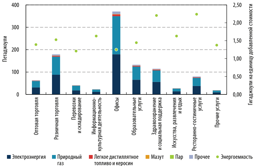
Рисунок 4.3 • Пример разных уровней энергоемкости в Канаде, 2010 год
