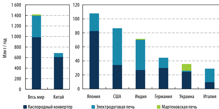
Рисунок 5.8 • Объемы производства по технологическим подходам и энергоёмкость для отдельных стран, 2010 год
