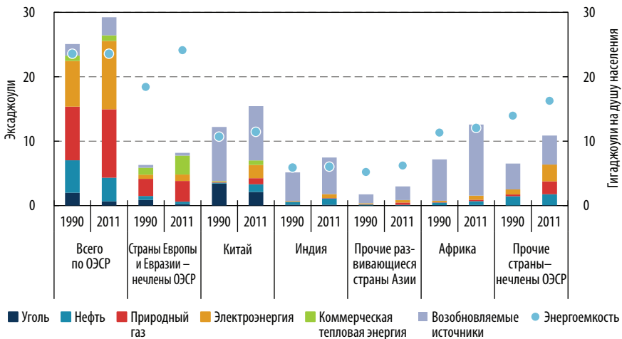
Рисунок 3.2 • Энергопотребление и совокупная энергоемкость жилищного сектора
