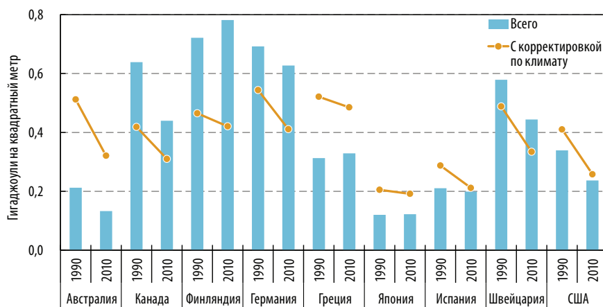
Рисунок 3.8 • Энергоемкость отопления с корректировкой по климату и без нее
