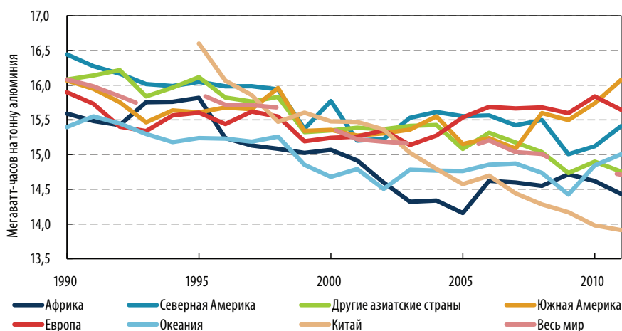
Рисунок 5.12 • Удельное потребление электроэнергии при выплавке алюминия по регионам
