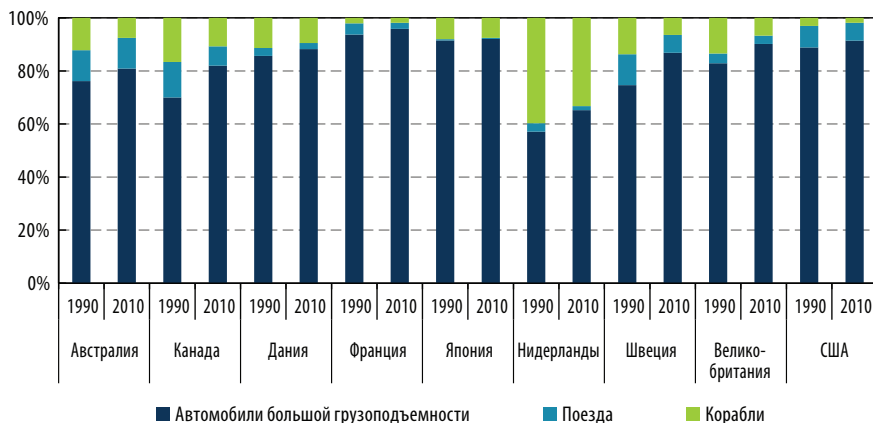
Рисунок 6.11 • Энергопотребление по видам грузового транспорта
