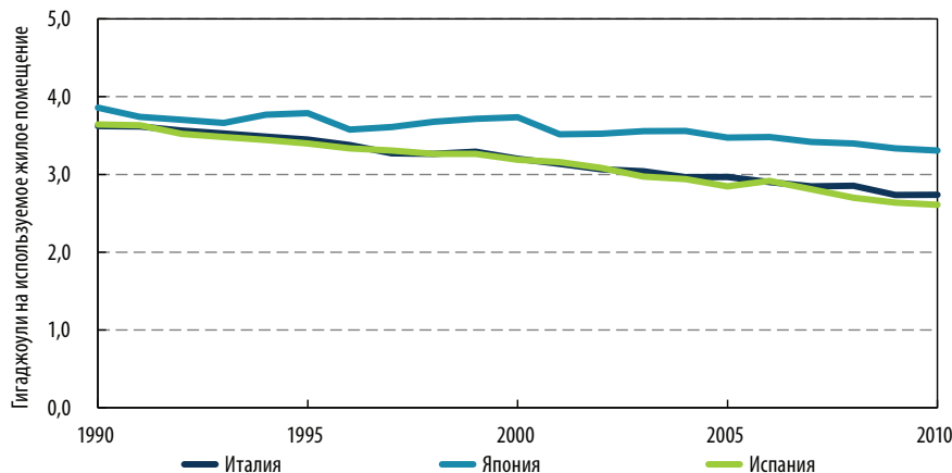
Рисунок 3.12 • Примеры энергоемкости процессов приготовления пищи в отдельных странах (энергия на используемое жилое помещение)
