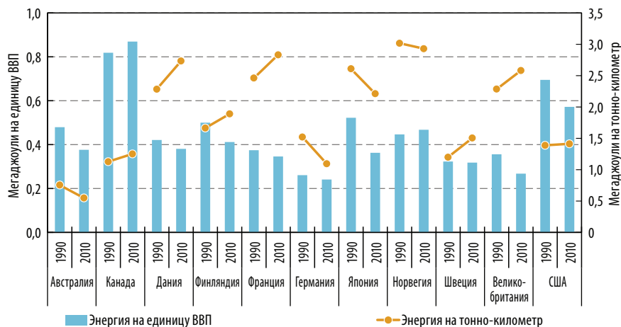
Рисунок 6.15 • Пример показателя уровня 1 для отдельных стран: энергоёмкость грузового транспорта
