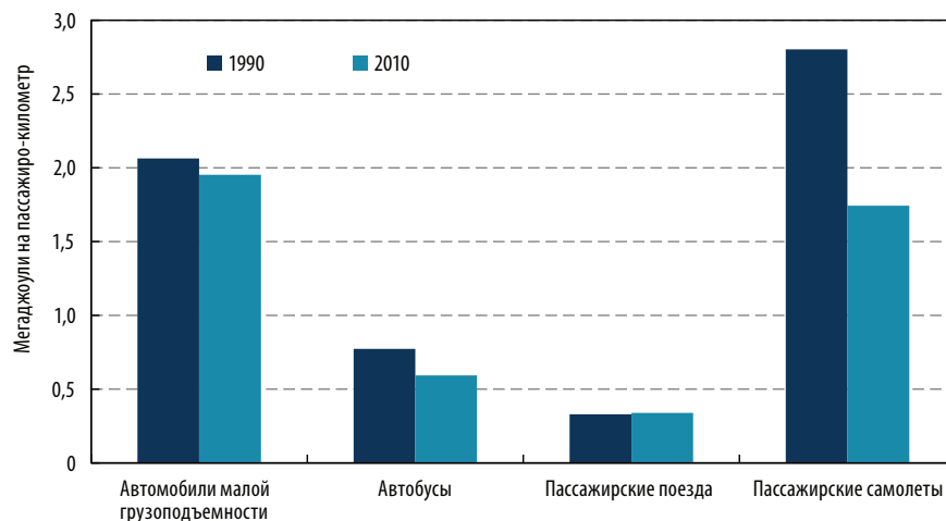
Рисунок 6.7 • Пример показателей уровня 2 для стран МЭА15: энергопотребление на пассажиро-километр по видам транспорта
