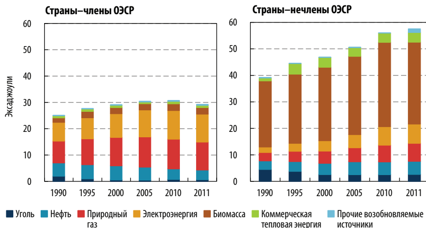
Рисунок 3.1 • Потребление энергии в жилищном секторе стран-членов ОЭСР и стран-нечленов ОЭСР
