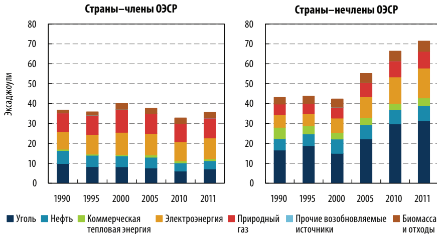
Рисунок 5.2 • Энергопотребление промышленности в странах-членах ОЭСР и странах-нечленах ОЭСР
