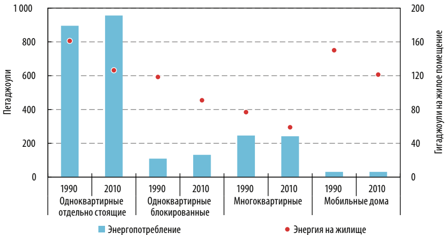
Рисунок 3.7 • Энергопотребление и энергоёмкость для разных видов жилья в Канаде
