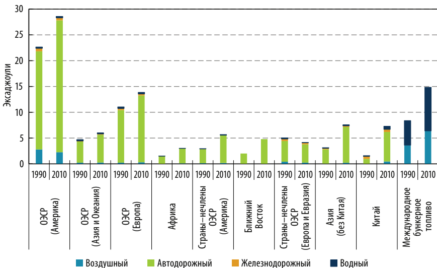
Рисунок 6.1 • Энергопотребление по видам транспорта
