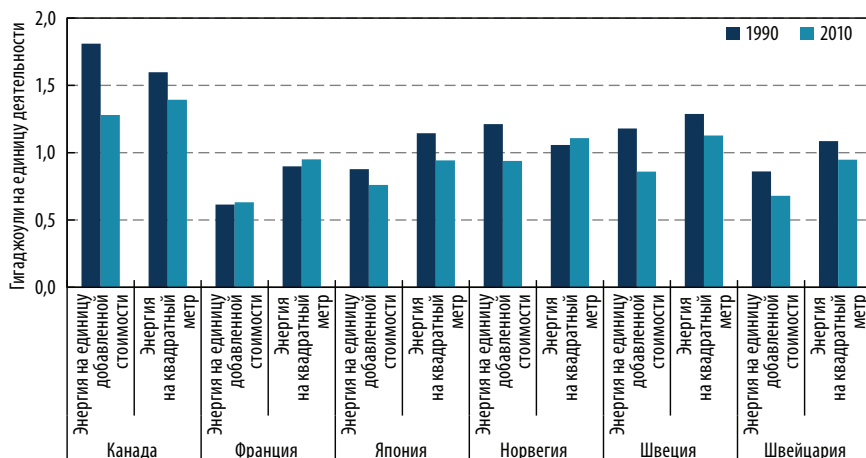
Рисунок 4.5 • Примеры показателей уровня 1 в отдельных странах
