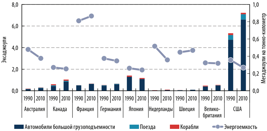
Рисунок 6.12 • Энергопотребление и энергоёмкость грузового транспорта
