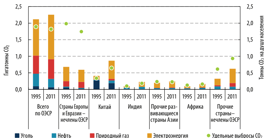
Рисунок 3.3 • Выбросы и удельные показатели CO 2 для жилищного сектора
