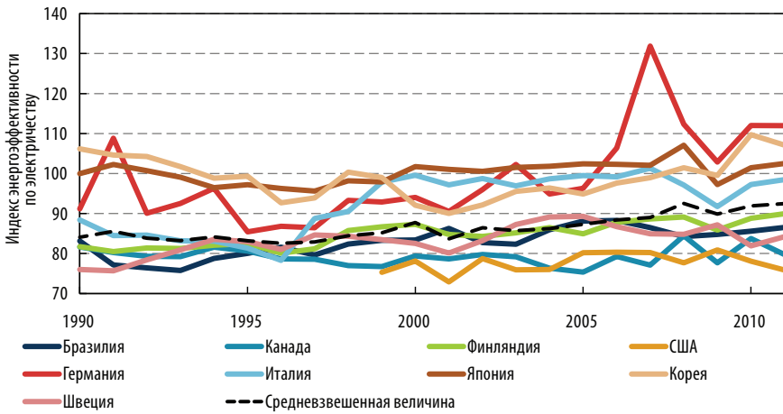
Рисунок 5.10 • Потенциал эффективного использования электроэнергии
