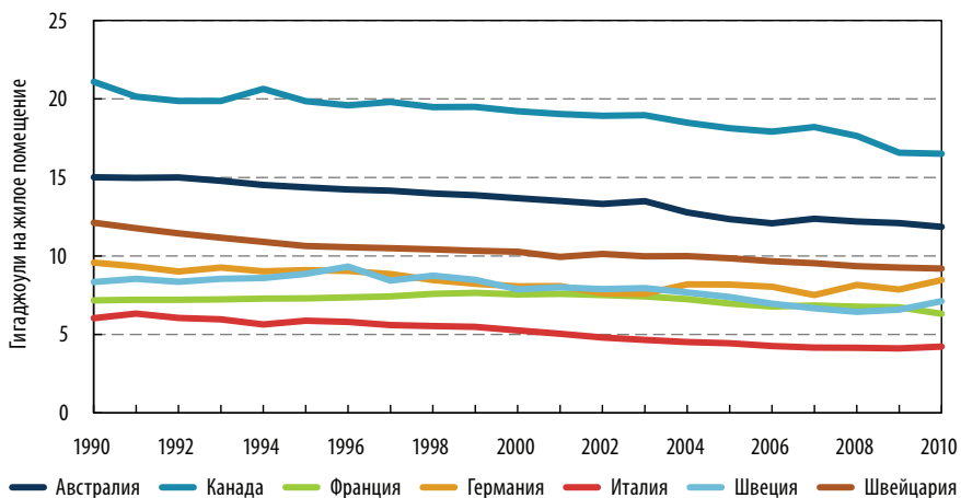
Рисунок 3.9 • Примеры энергоемкости горячего водоснабжения в различных странах (энергопотребление на используемое жилое помещение)
