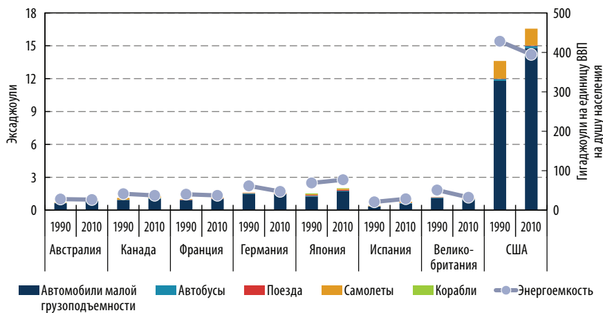
Рисунок 6.3 • Энергопотребление пассажирского транспорта в абсолютных величинах и на единицу ВВП на душу населения
