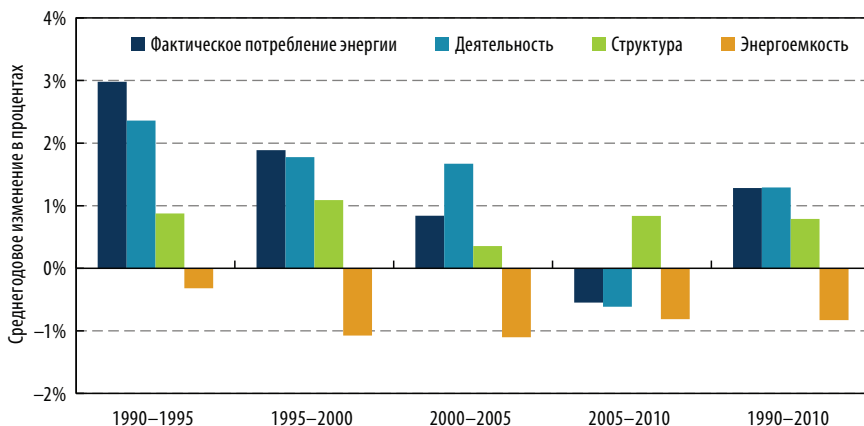
Рисунок 6.18 • Факторы, влияющие на энергопотребление грузового транспорта в странах МЭА15
