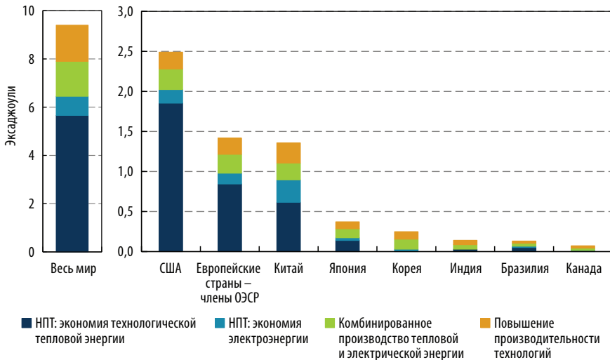
Рисунок 5.11 • Текущий потенциал экономии энергии для химии и нефтехимии на основе НДТ, 2010 год
