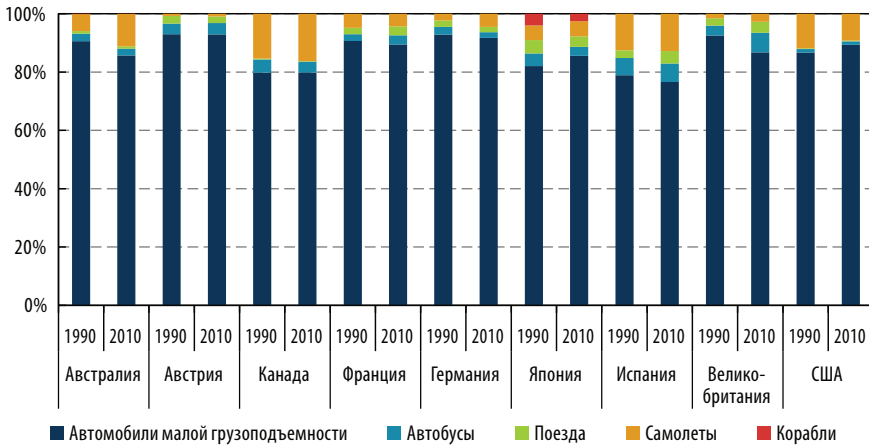
Рисунок 6.2 • Энергопотребление по видам пассажирского транспорта для разных стран
