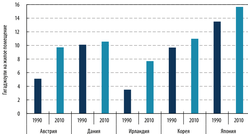
Рисунок 3.13 • Примеры энергоемкости бытовой техники в отдельных странах (энергия на используемое жилое помещение)
