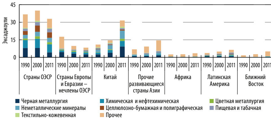
Рисунок 5.3 • Энергопотребление по подсекторам промышленности
