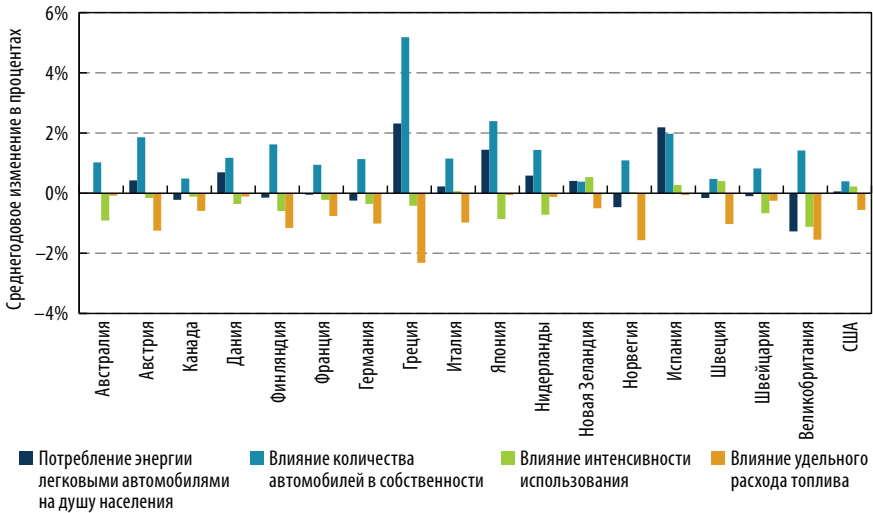
Рисунок 6.10 • Декомпозиция изменений в энергопотреблении АМГ на душу населения, 1990–2010 годы
