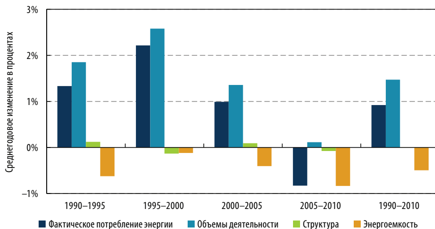
Рисунок 6.9 • Факторы, влияющие на энергопотребление пассажирского транспорта в странах МЭА15
