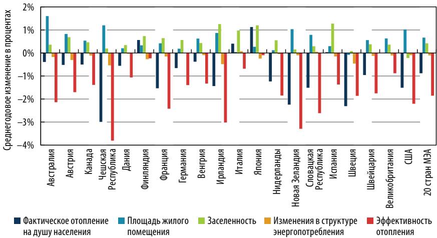
Рисунок 3.15 • Декомпозиция изменений в энергопотреблении для отопления на душу населения, 1990–2010 годы
