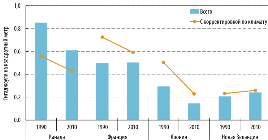
Рисунок 4.6 • Наблюдаемая и скорректированная по климату энергоемкость для отдельных стран
