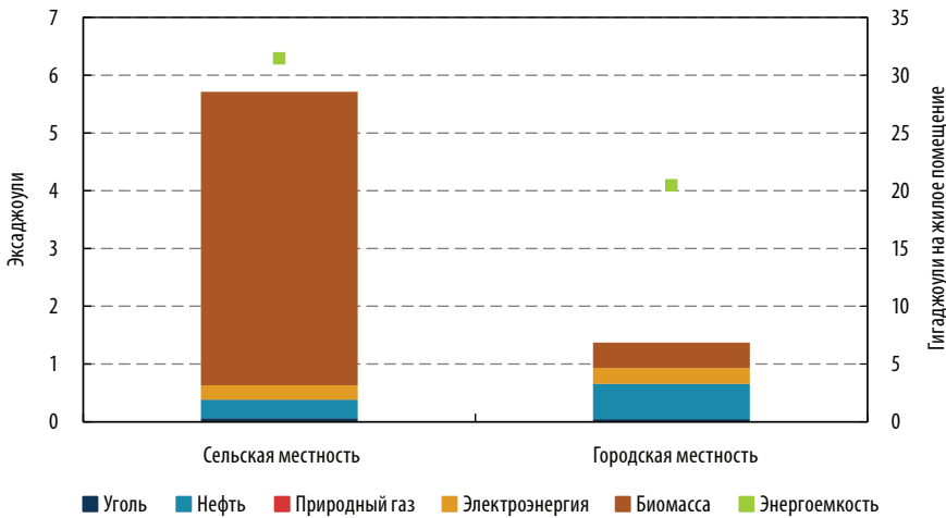
Рисунок 3.6 • Оценка энергопотребления и энергоемкости в сельской и городской местности Индии в 2010 году
