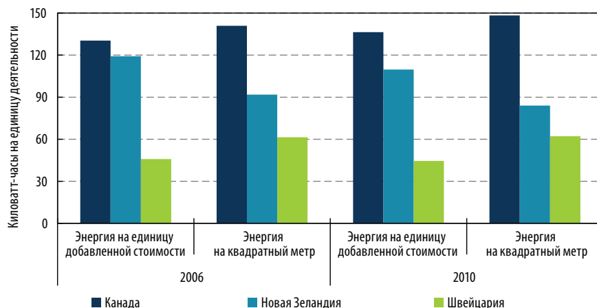
Рисунок 4.8 • Примеры энергоёмкости в категории прочего оборудования для отдельных стран
