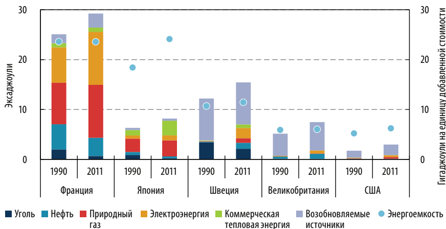
Рисунок 4.2 • Энергопотребление и совокупная энергоемкость сектора услуг
