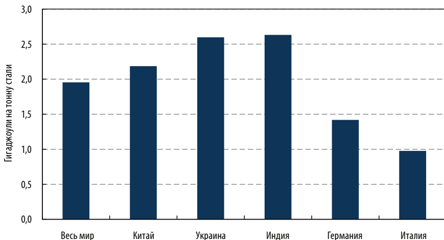
Рисунок 5.7 • Энергопотребление в черной и цветной металлургии на тонну произведенной страной стали в 2010 году
