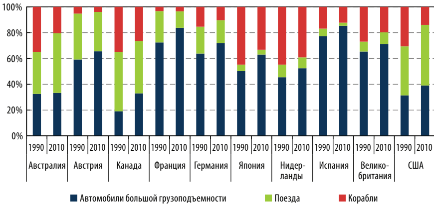
Рисунок 6.13 • Доля видов транспорта в общих тонно-километрах
