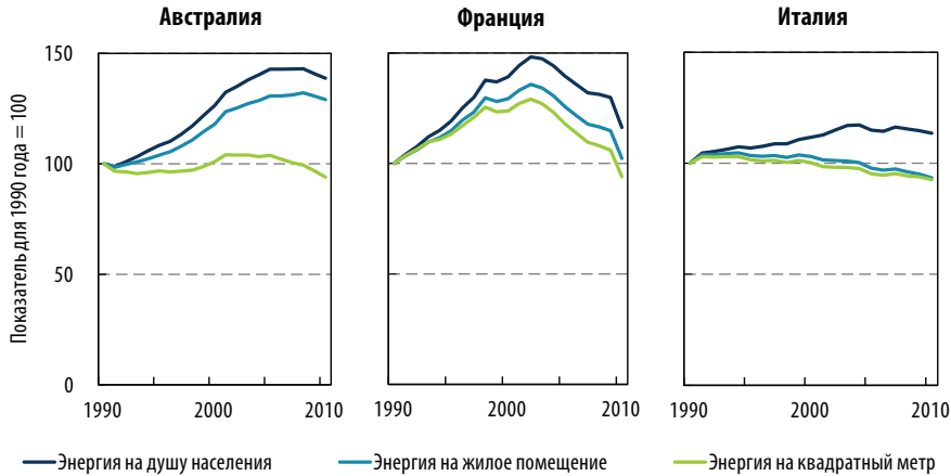
Рисунок 3.11 • Примеры энергоёмкости в Австралии, Франции и Италии
