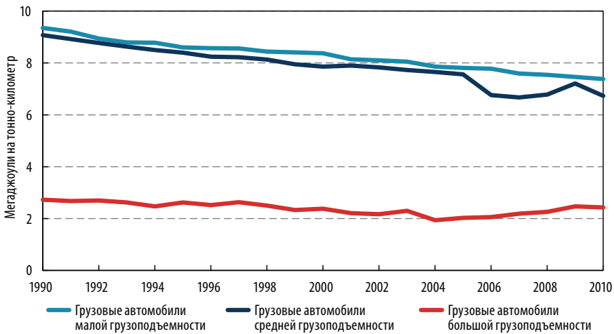
Рисунок 6.17 • Тенденции энергоемкости для разных типов автомобилей: пример Канады
