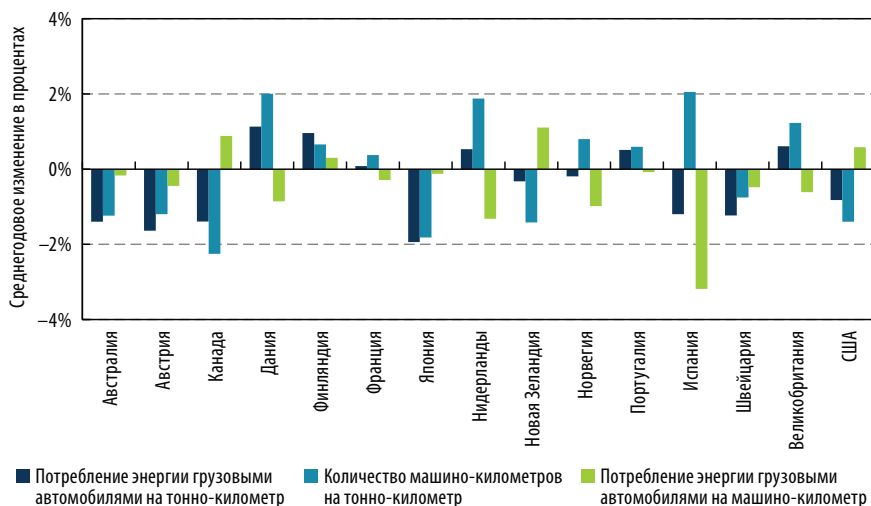
Рисунок 6.19 • Декомпозиция изменений в энергоёмкости грузовых автомобилей в странах МЭА15, 1990–2010 годы
